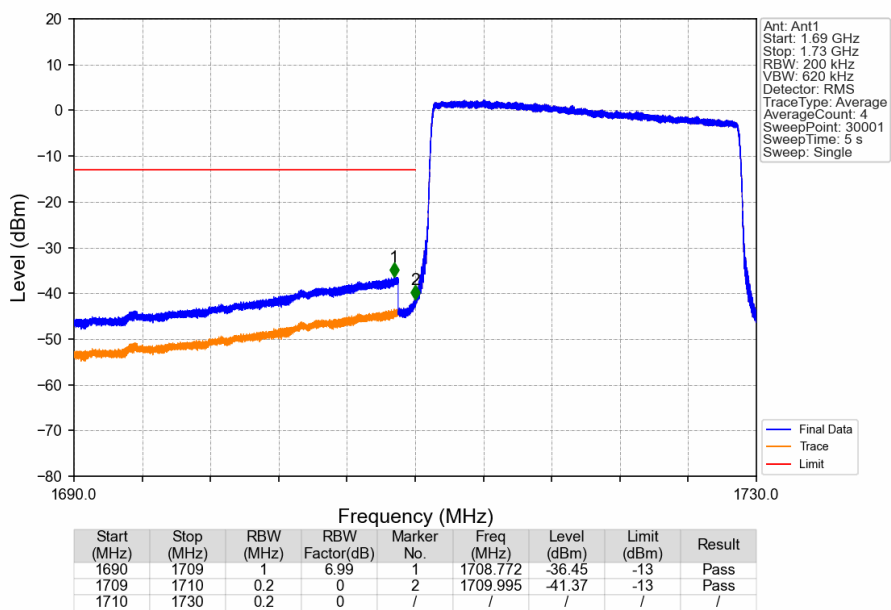
Band4_20MHz_16QAM_LCH_1720MHz_RB_100_0_NTNV
