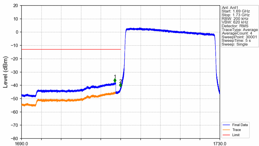
Band4_20MHz_QPSK_LCH_1720MHz_RB_100_0_NTNV
