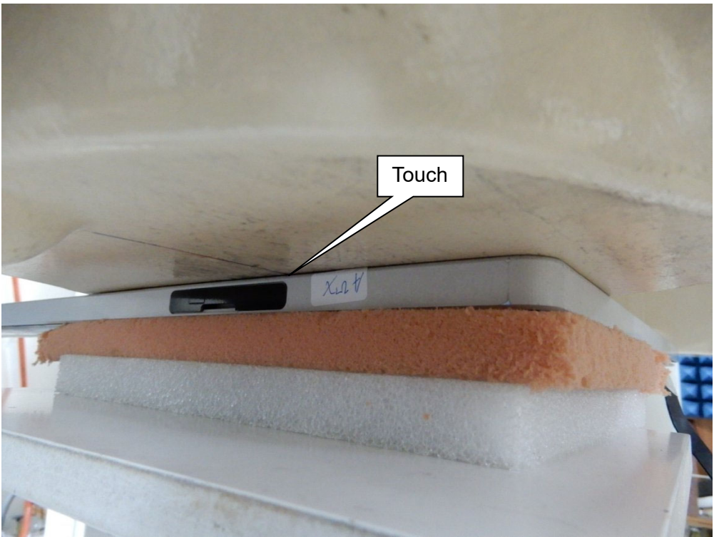
EUT Back – Limb SAR (Aux Antenna)
