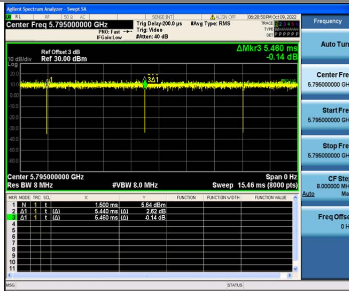
802.11ax(HE40)_Ant2_5795
