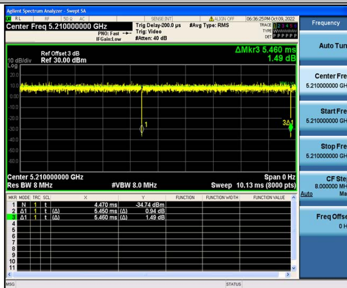
802.11ax(HE80)_Ant2_5210
