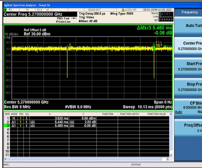
802.11ax(HE40)_Ant2_5270
