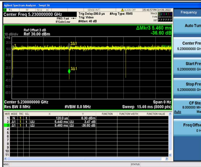
802.11ax(HE40)_Ant2_5230
