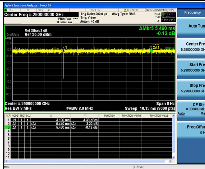
802.11ax(HE80)_Ant2_5290
