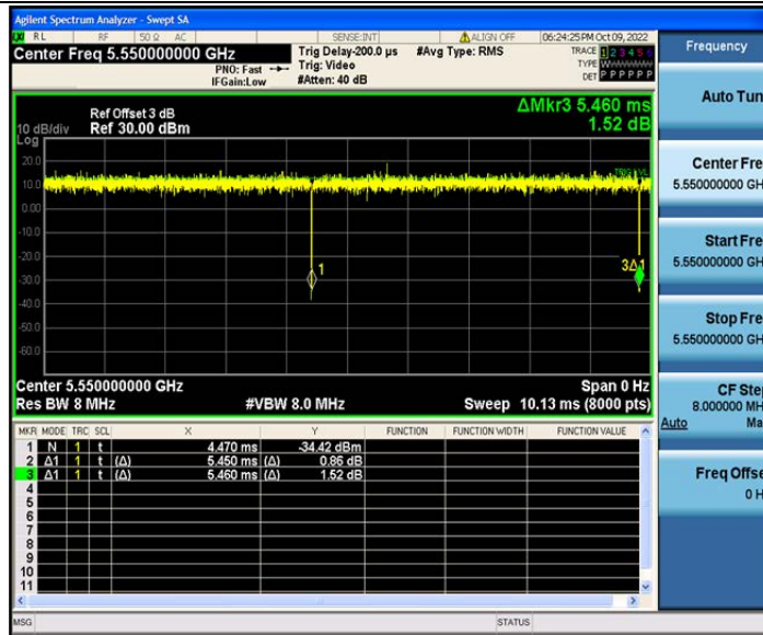
802.11ax(HE40)_Ant2_5550
