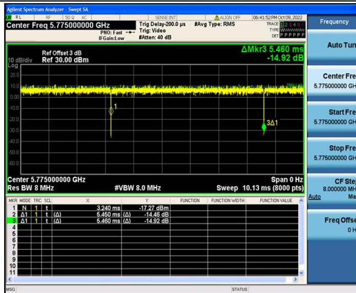
802.11ax(HE80)_Ant2_5775
