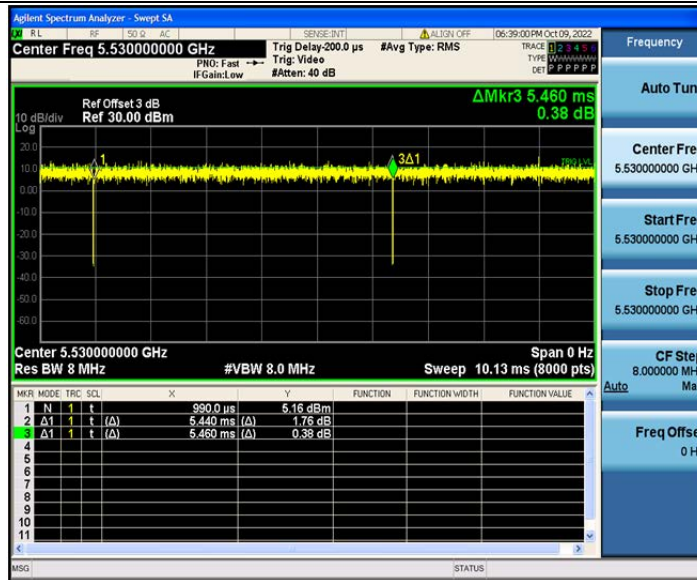
802.11ax(HE80)_Ant2_5530
