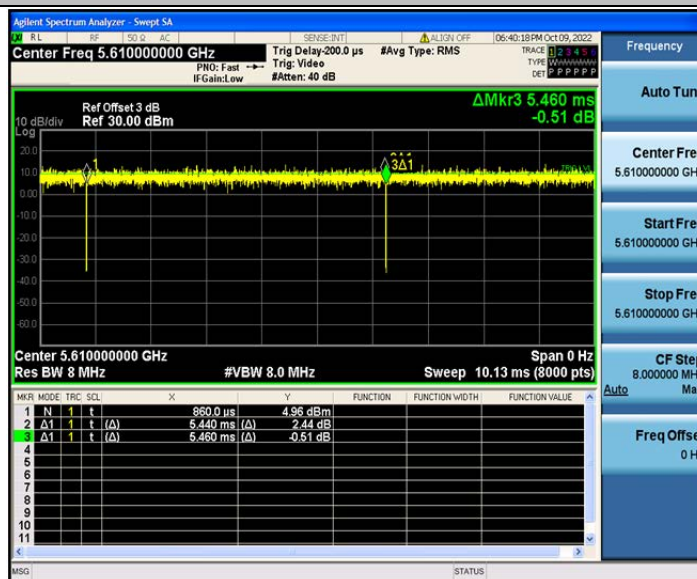
802.11ax(HE80)_Ant2_5610
