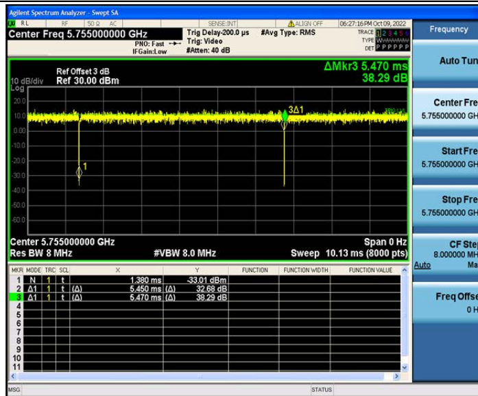
802.11ax(HE40)_Ant2_5755
