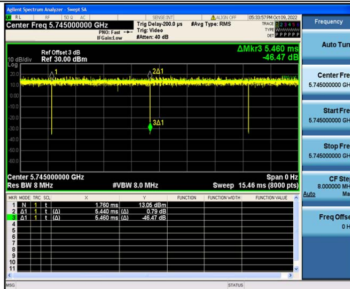
802.11ax(HE20)_Ant2_5745
