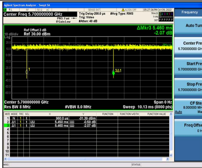
802.11ax(HE20)_Ant2_5700
