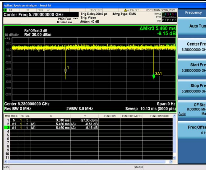
802.11ax(HE20)_Ant2_5280
