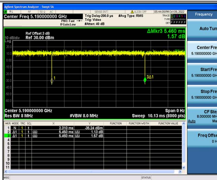
802.11ax(HE40)_Ant2_5190
