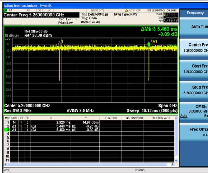
802.11ax(HE20)_Ant2_5260
