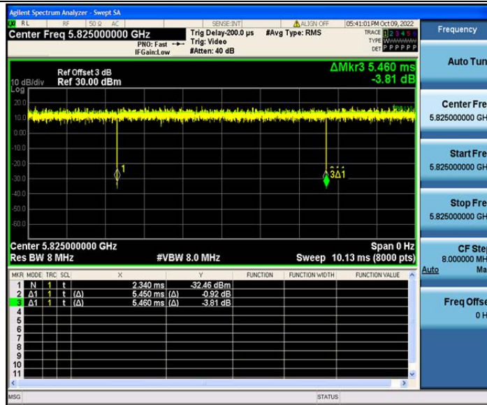
802.11ax(HE20)_Ant2_5825
