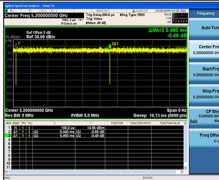
802.11ax(HE20)_Ant2_5200
