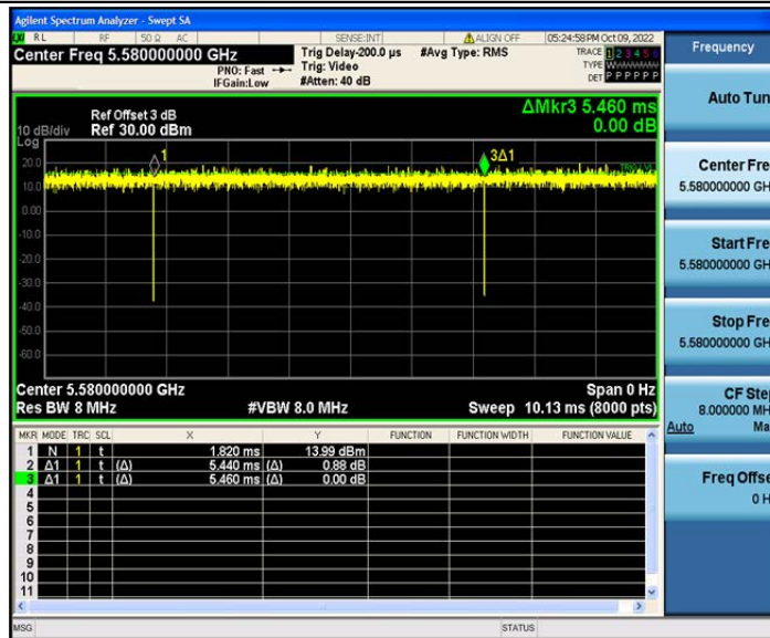
802.11ax(HE20)_Ant2_5580
