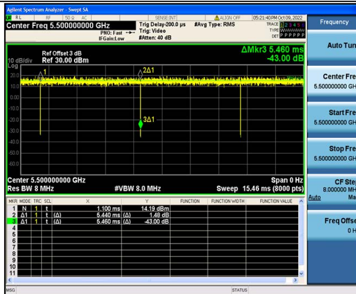
802.11ax(HE20)_Ant2_5500
