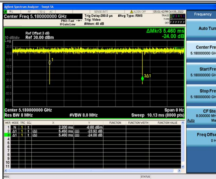
802.11ax(HE20)_Ant2_5180
