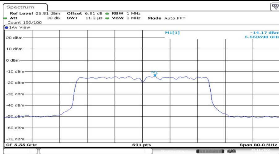
802.11ax(HE40)_Ant2_5550 242/61
