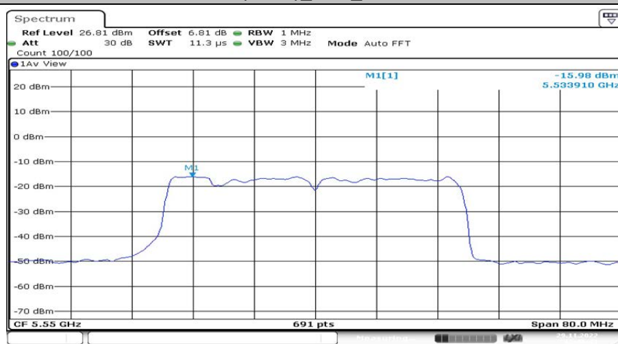
802.11ax(HE40)_Ant2_5550 242/61
