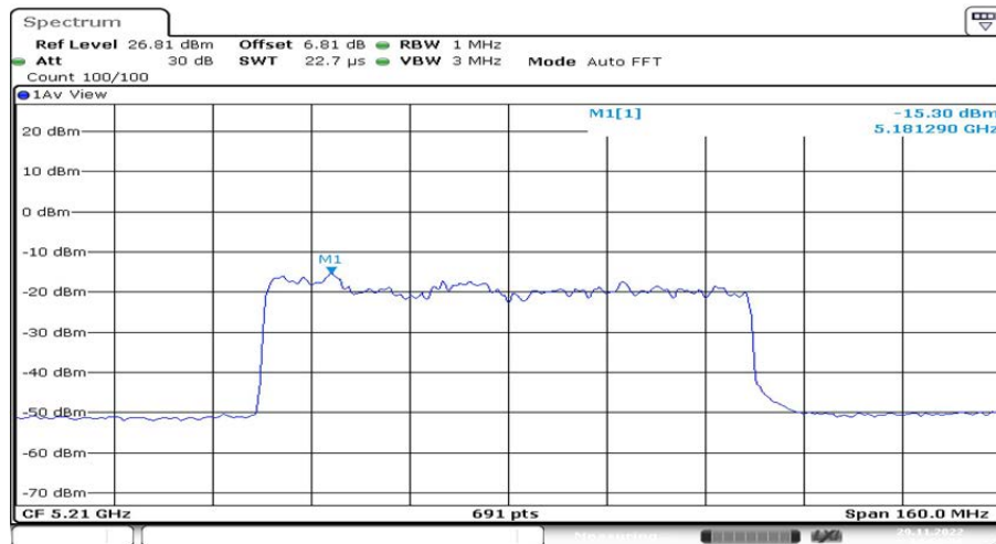
802.11ax(HE80)_Ant1_5210 242/62
