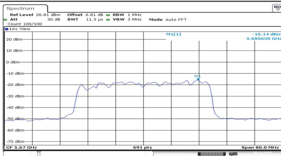
802.11ax(HE40)_Ant1_5670 242/61
