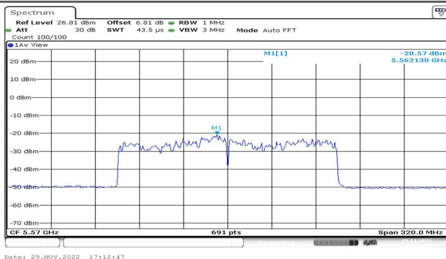
802.11ax(HE160)_Ant2_5570 242/64
