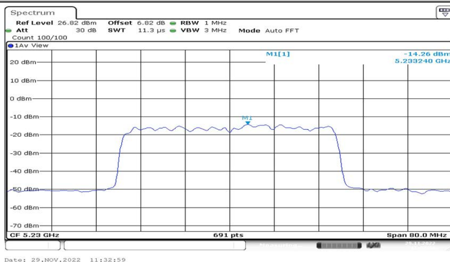
802.11ax(HE40)_Ant2_5230 242/61
