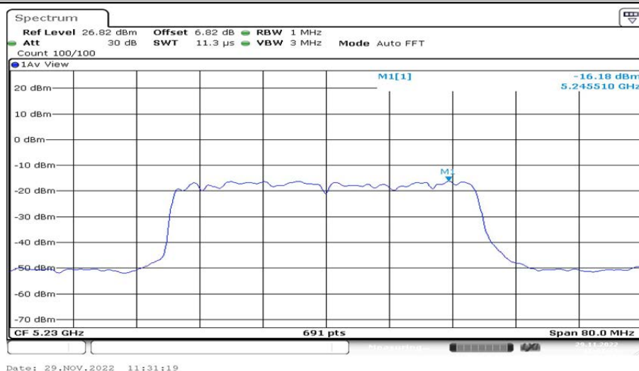
802.11ax(HE40)_Ant2_5230 106/54
