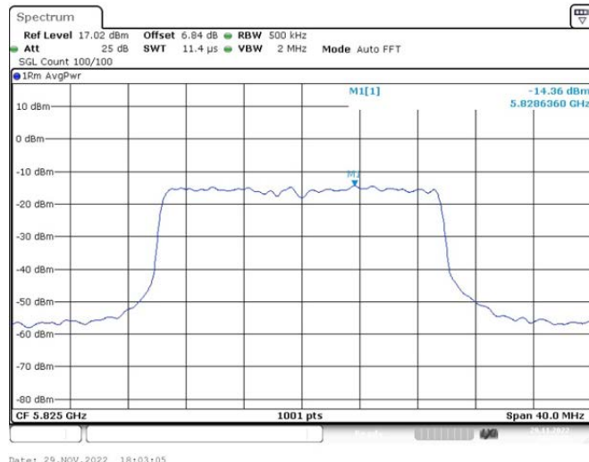
802.11ax(HE20)_Ant2_5825 52/38
