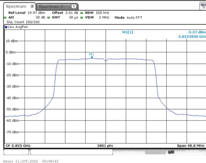
802.11ax(HE20)_Ant2_5825 242/61
