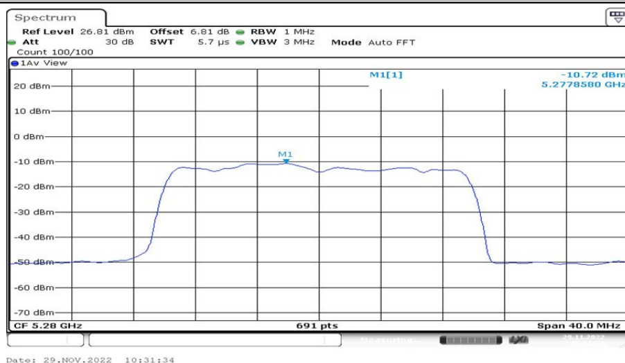
802.11ax(HE20)_Ant2_5280 52/38
