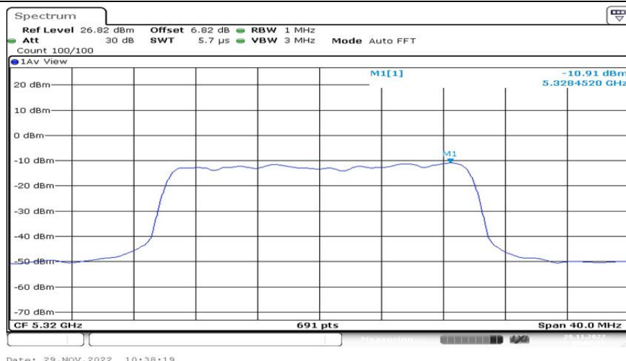
802.11ax(HE20)_Ant2_5320 52/38
