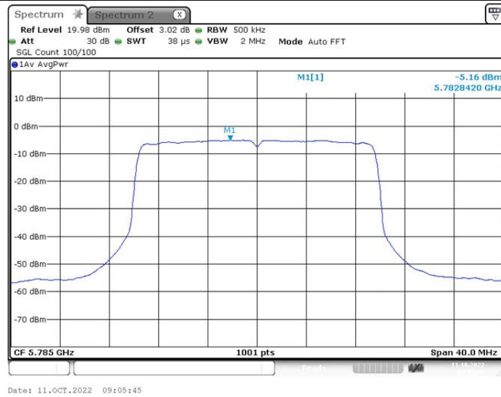
802.11ax(HE20)_Ant2_5785 242/61
