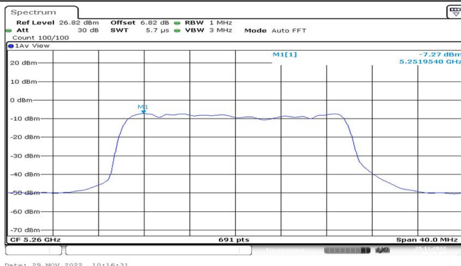
802.11ax(HE20)_Ant2_5260 52/38
