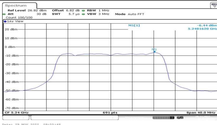
802.11ax(HE20)_Ant2_5240 52/38
