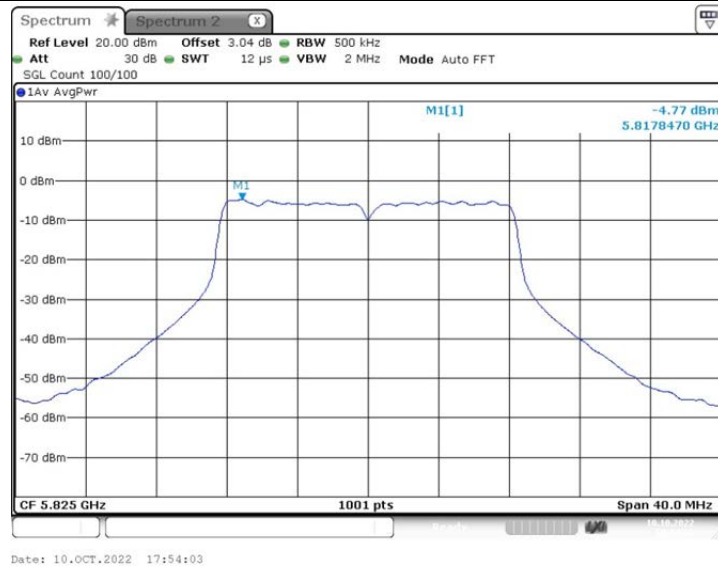
802.11a_Ant2_5825
