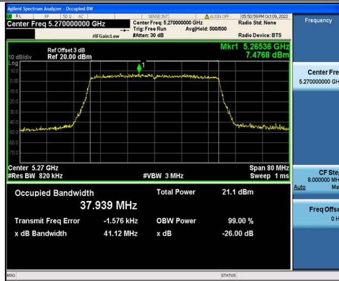
802.11ax(HE40)_Ant2_5270 484/65
