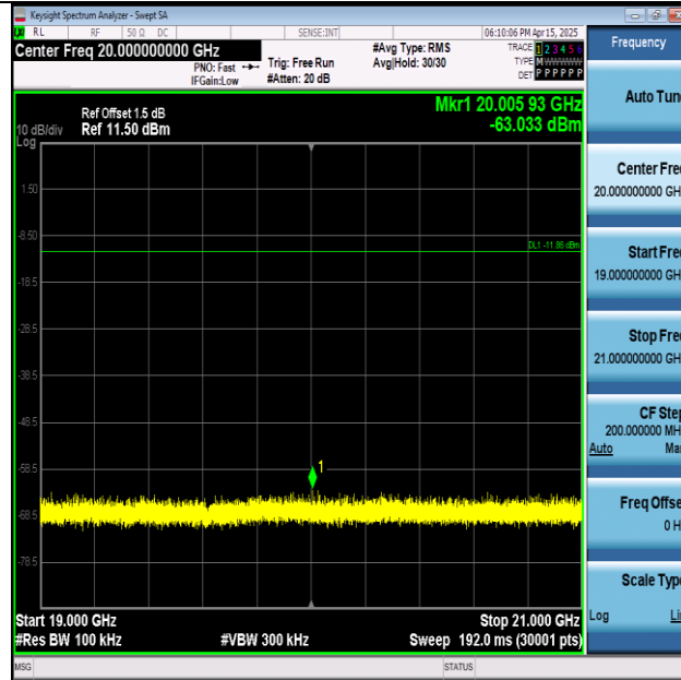
11N20SISO-Ant1-2462-19000~21000-PASS
