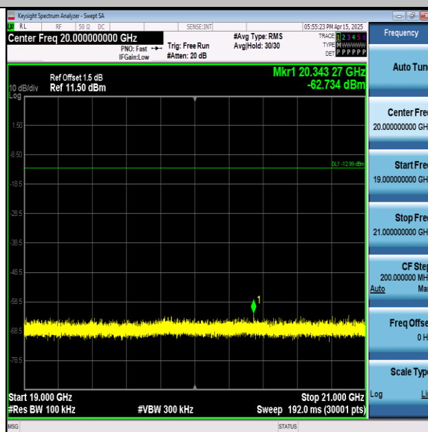
11G-Ant1-2462-19000~21000-PASS
