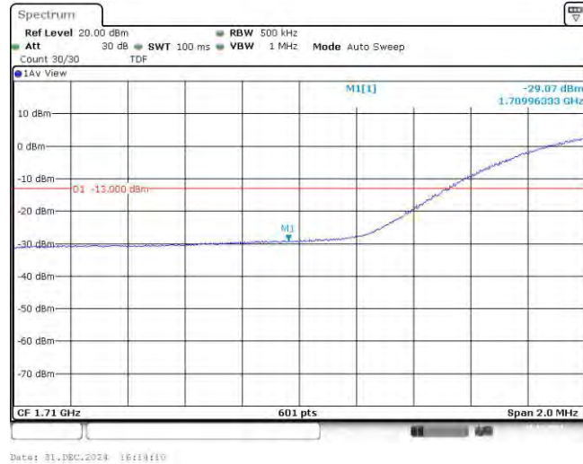
Band66-20MHz-QPSK-132572-100RB#0
