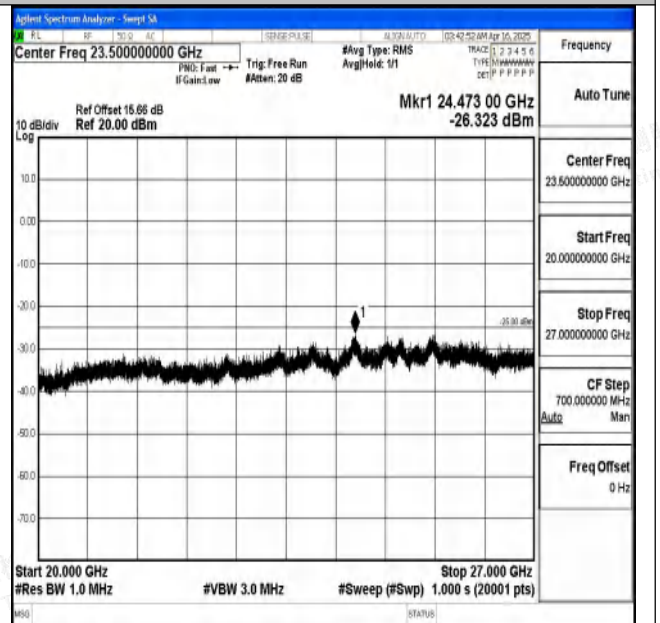
Band7_20MHz_16QAM_20850_1RB#0_20000~27000_200 00~27000
