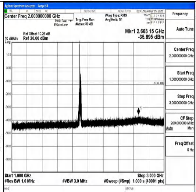
Band2-20MHz-QPSK-19100-1RB#0-1000~3000-PASS
