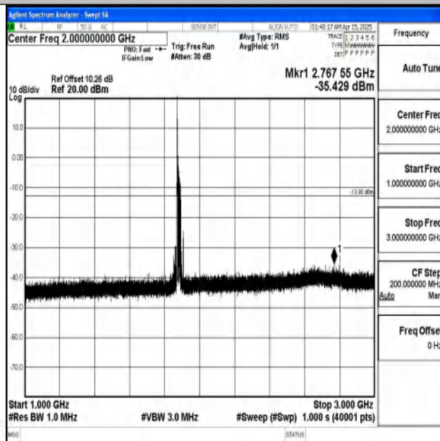
Band2-20MHz-QPSK-18900-1RB#0-1000~3000-PASS
