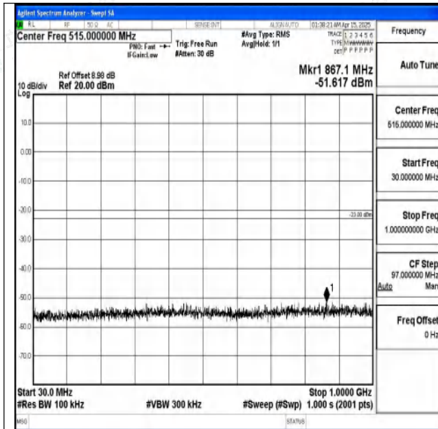
Band2-20MHz-QPSK-18700-1RB#0-30~1000-PASS
