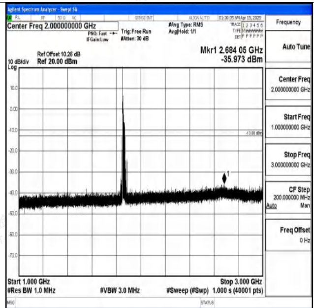
Band2-20MHz-QPSK-18700-1RB#0-1000~3000-PASS
