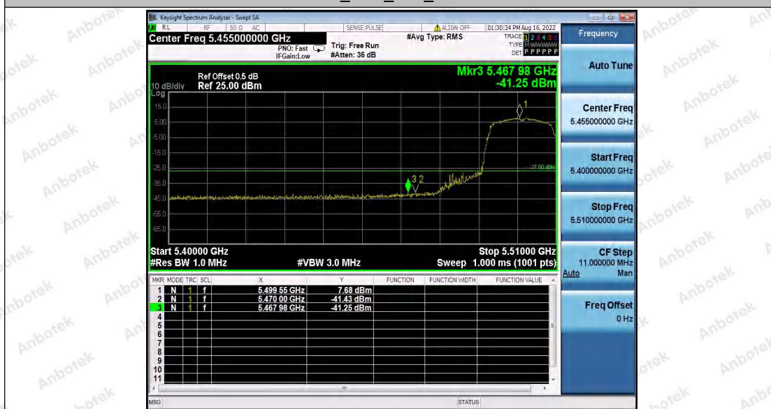
11A_Ant1_Low_5500
