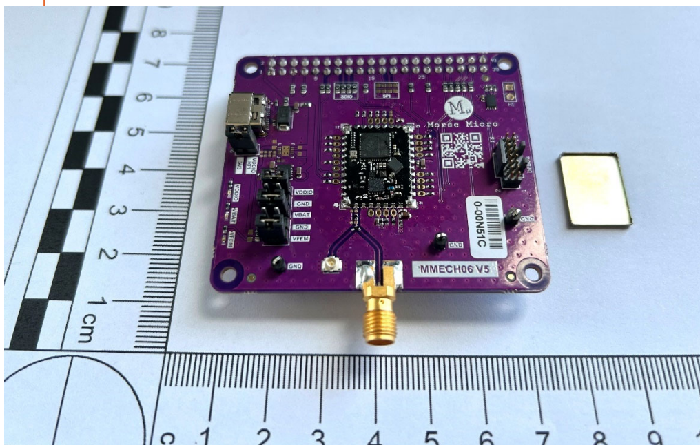
RFIC
