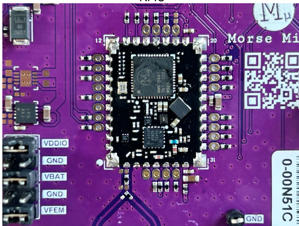
RFIC
