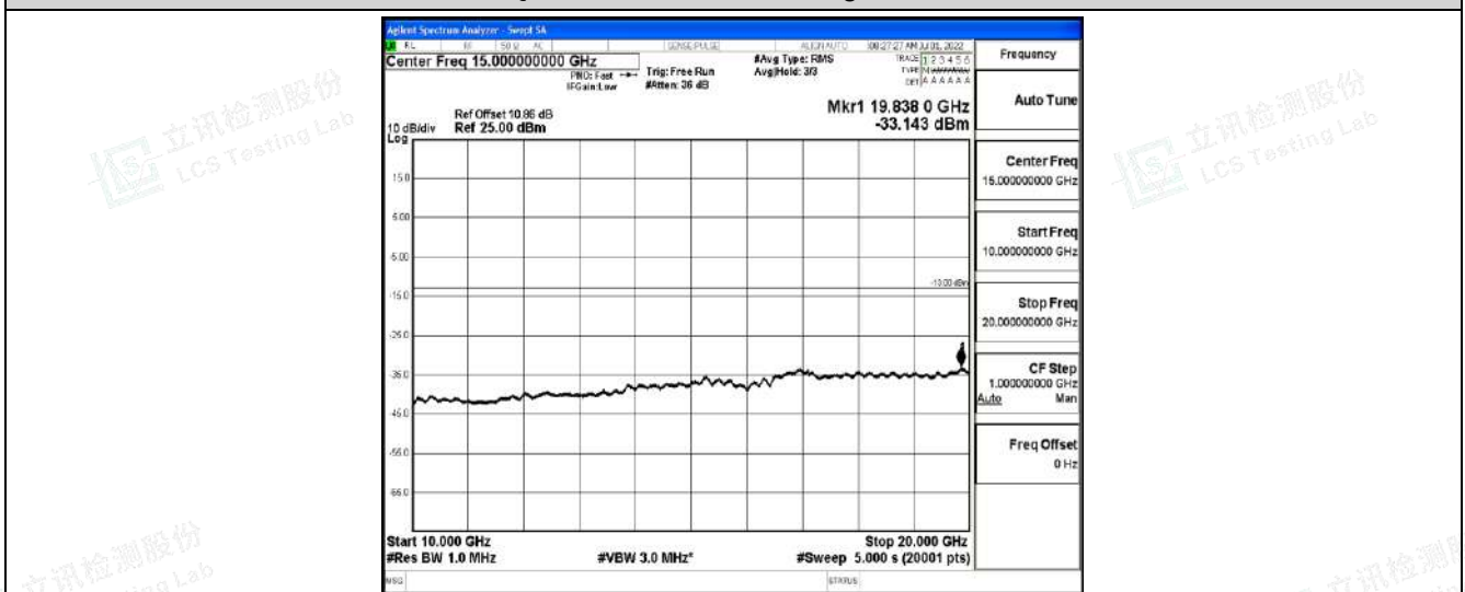
Band4-3MHz-QPSK-20175-1RB#0-Range5:10000~20000MHz
