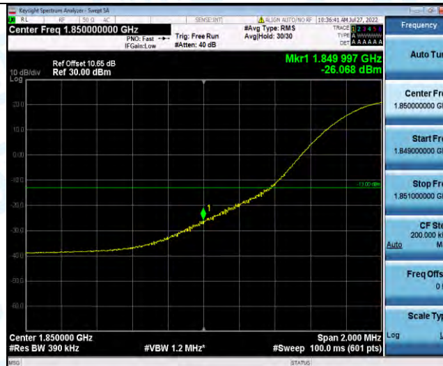
Band2-20MHz-QPSK-18700-1RB#99
