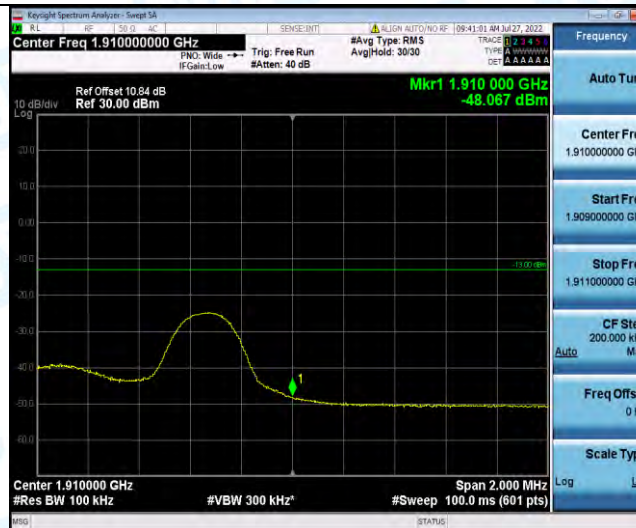
Band2-5MHz-QPSK-19175-1RB#24
