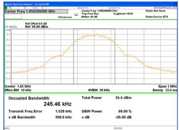
GPRS1900_Low
