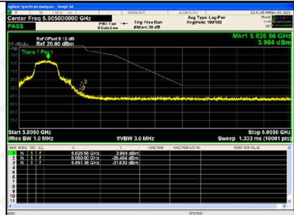
802.11(n20)-5825
