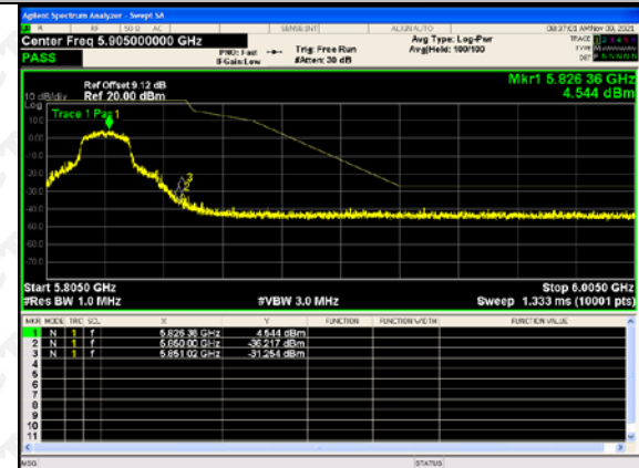
802.11(n20)-5825
