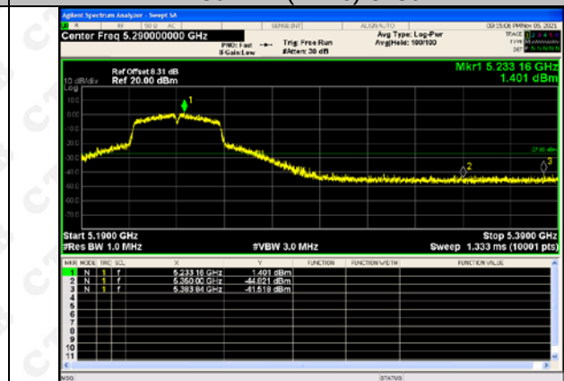
802.11n(HT40)-5230
