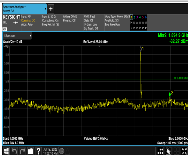
Band4-3MHz-QPSK-20175-1RB#0-Range2:1000~2000MHz
