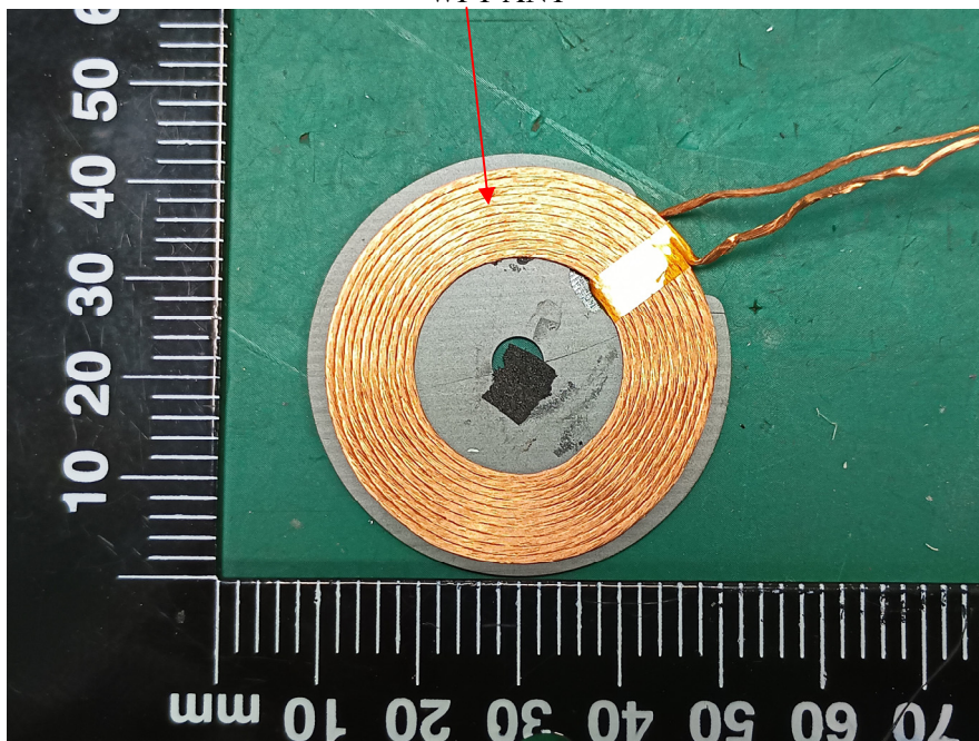
WPT ANT
