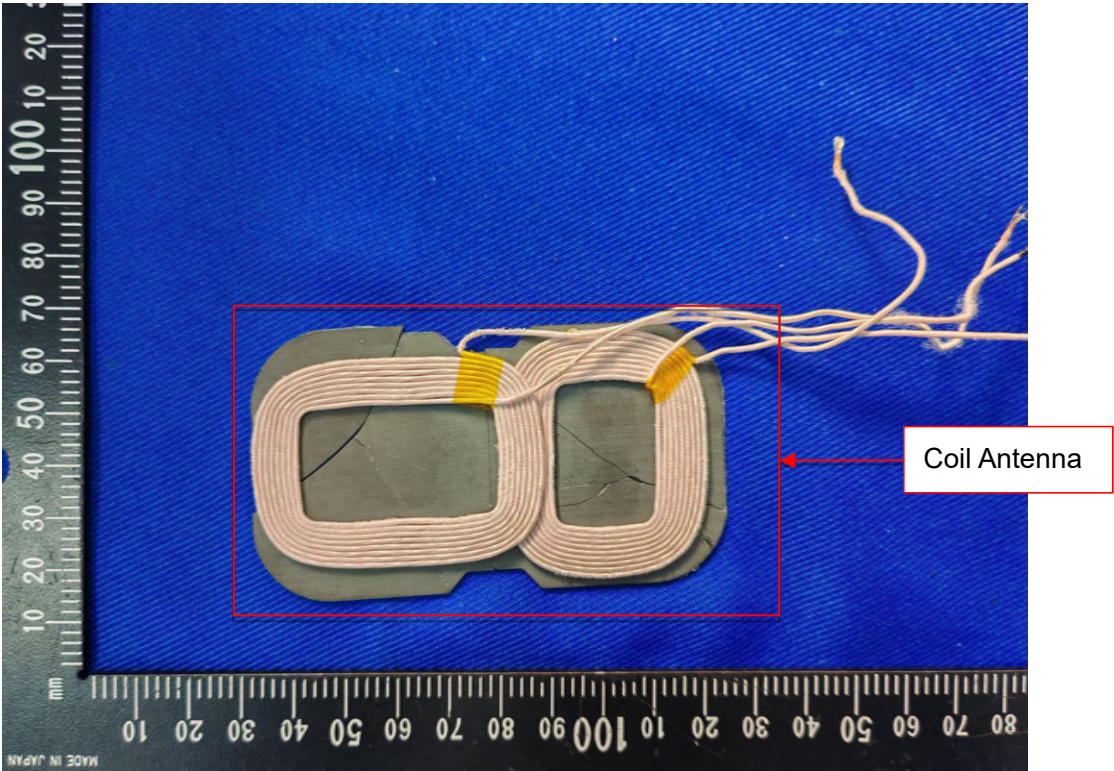
EUT Photo
