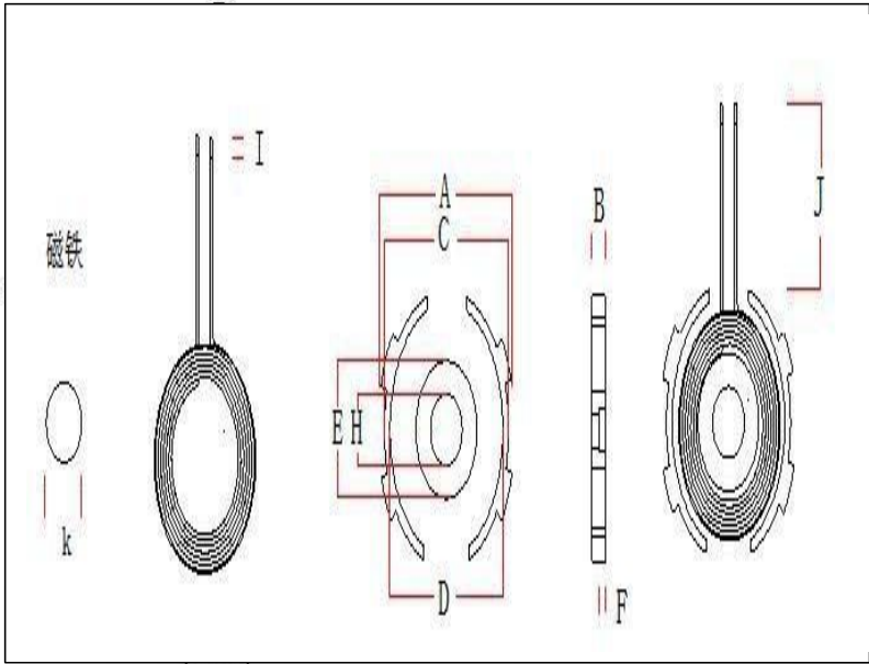
一、尺寸 DIMENSION:(mm)
