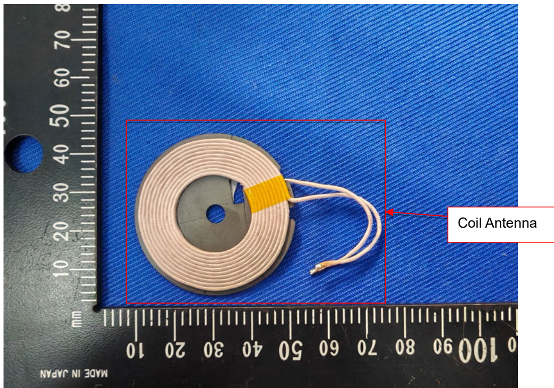
EUT Photo
