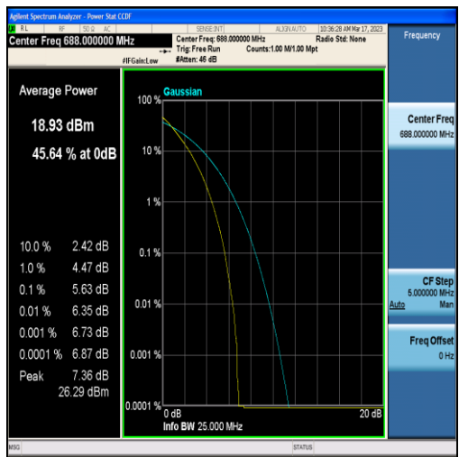
Band71-20MHz-QPSK-133372-100RB#0
