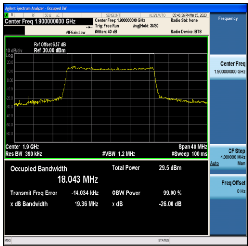
Band2-20MHz-QPSK-19100-100RB#0-18.043
