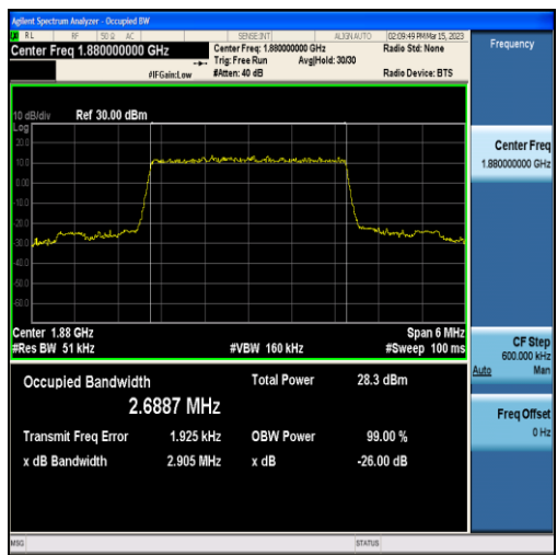
Band2-3MHz-QPSK-18900-15RB#0-2.6887
