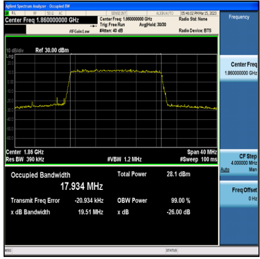
Band2-20MHz-16QAM-18700-100RB#0-17.934
