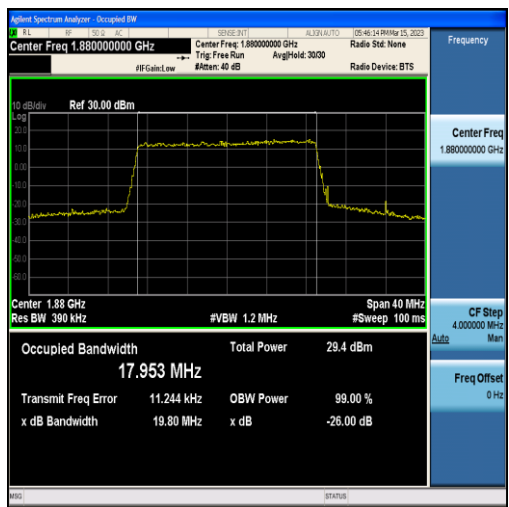
Band2-20MHz-QPSK-18900-100RB#0-17.953
