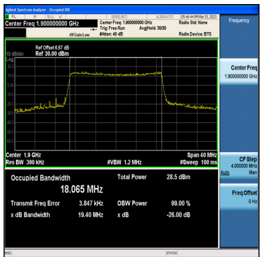
Band2-20MHz-16QAM-19100-100RB#0-18.065
