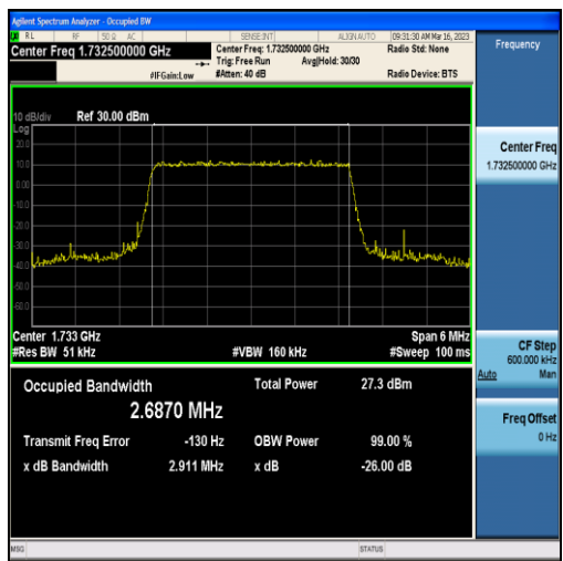
Band4-3MHz-QPSK-20175-15RB#0-2.6870
