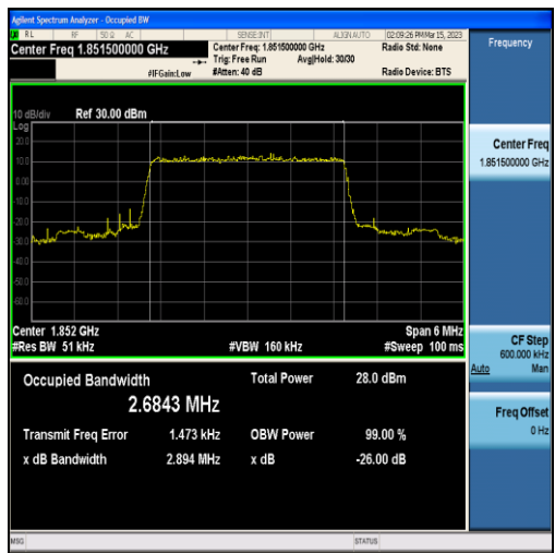
Band2-3MHz-QPSK-18615-15RB#0-2.6843
