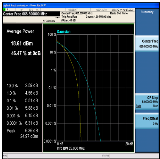
Band71-5MHz-QPSK-133147-25RB#0
