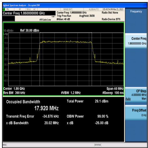
Band2-20MHz-QPSK-18700-100RB#0-17.920
