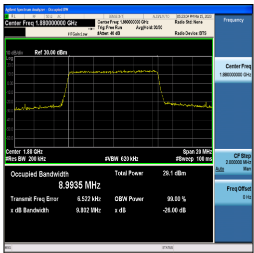
Band2-10MHz-QPSK-18900-50RB#0-8.9935
