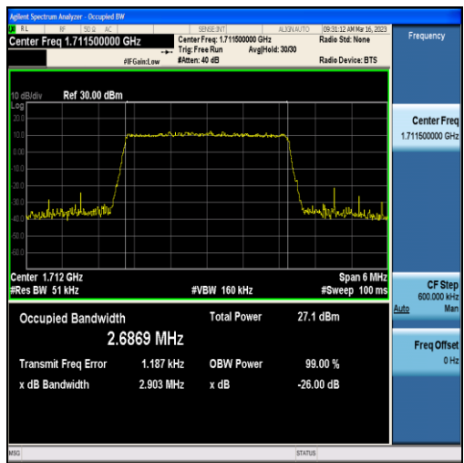
Band4-3MHz-QPSK-19965-15RB#0-2.6869
