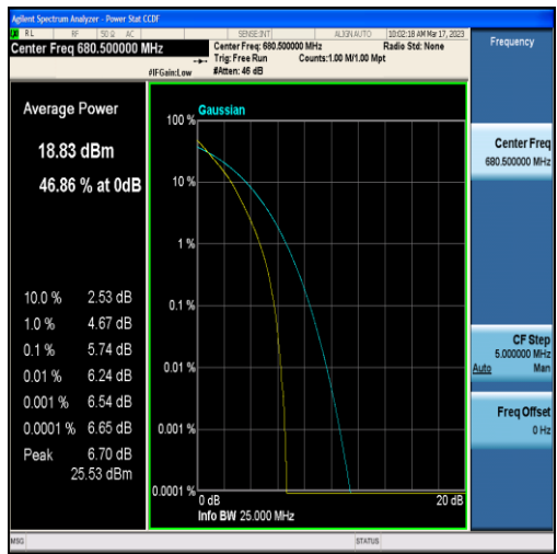
Band71-5MHz-QPSK-133297-25RB#0
