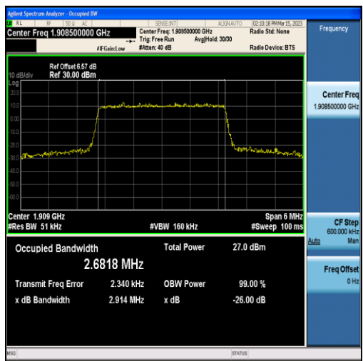
Band2-3MHz-16QAM-19185-15RB#0-2.6818
