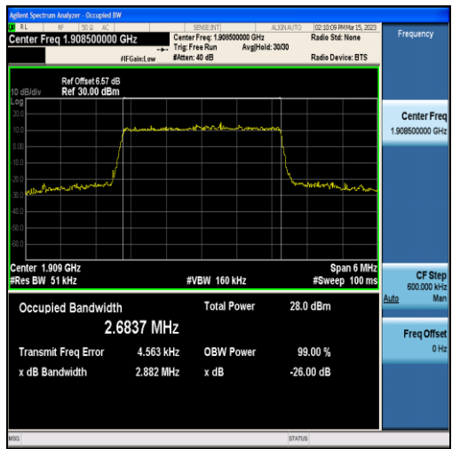
Band2-3MHz-QPSK-19185-15RB#0-2.6837
