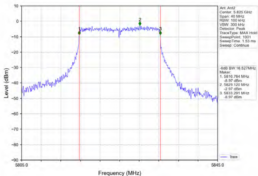
802.11a_HCH_5825MHz_Ant2_NTNV
