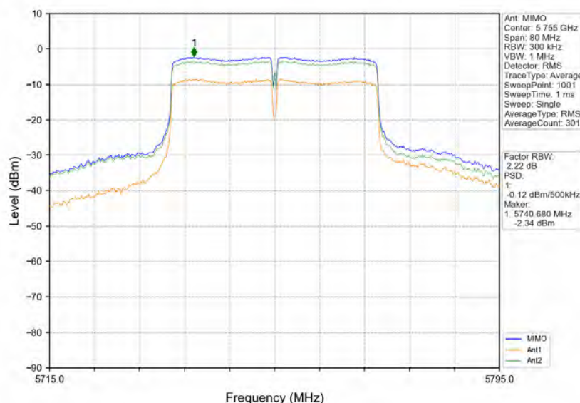
802.11n(HT40)_LCH_5755MHz_MIMO_NTNV
