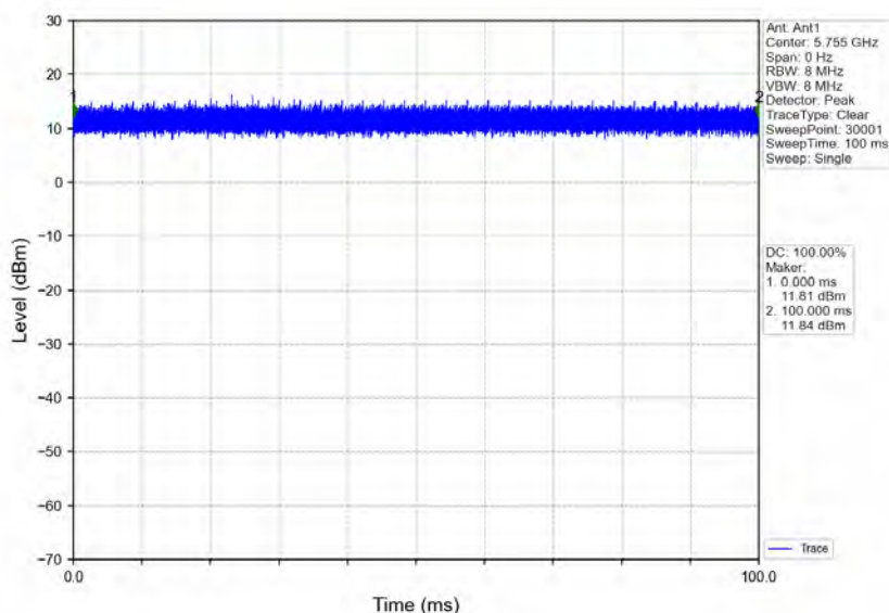
802.11ac(VHT40)_LCH_5755MHz_Ant1_NTNV
