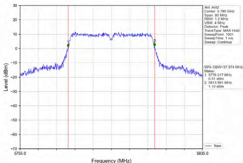
802.11n(HT40)_HCH_5795MHz_Ant2_NTNV
