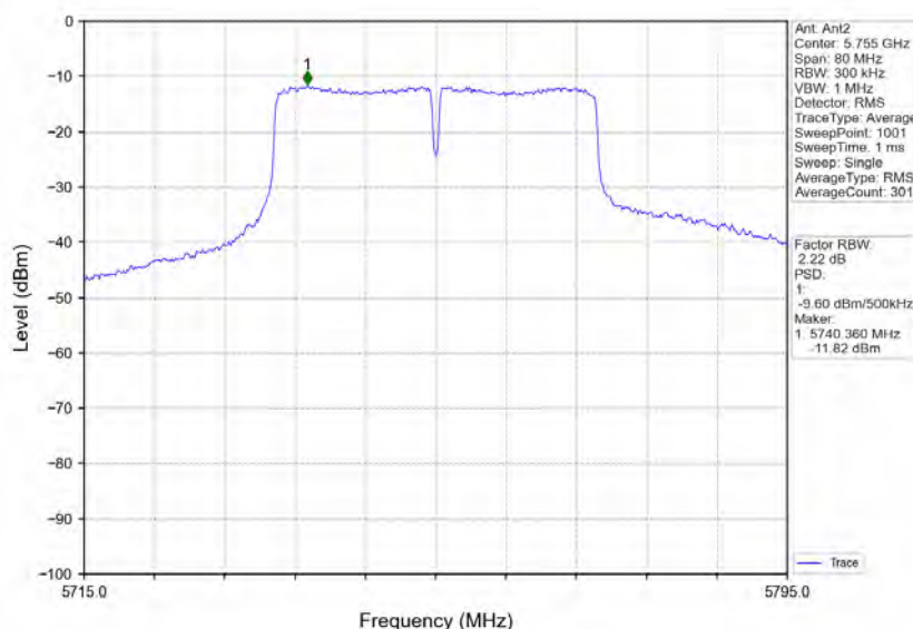
802.11ac(VHT40)_LCH_5755MHz_Ant2_NTNV
