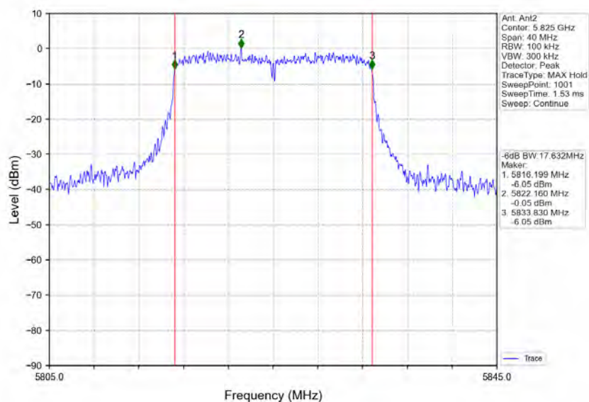
802.11n(HT20)_HCH_5825MHz_Ant2_NTNV
