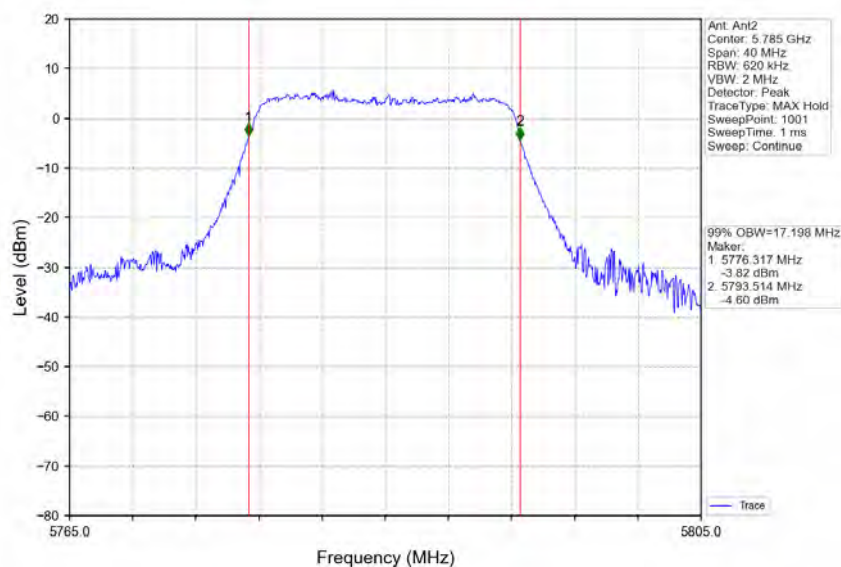
802.11a_MCH_5785MHz_Ant2_NTNV
