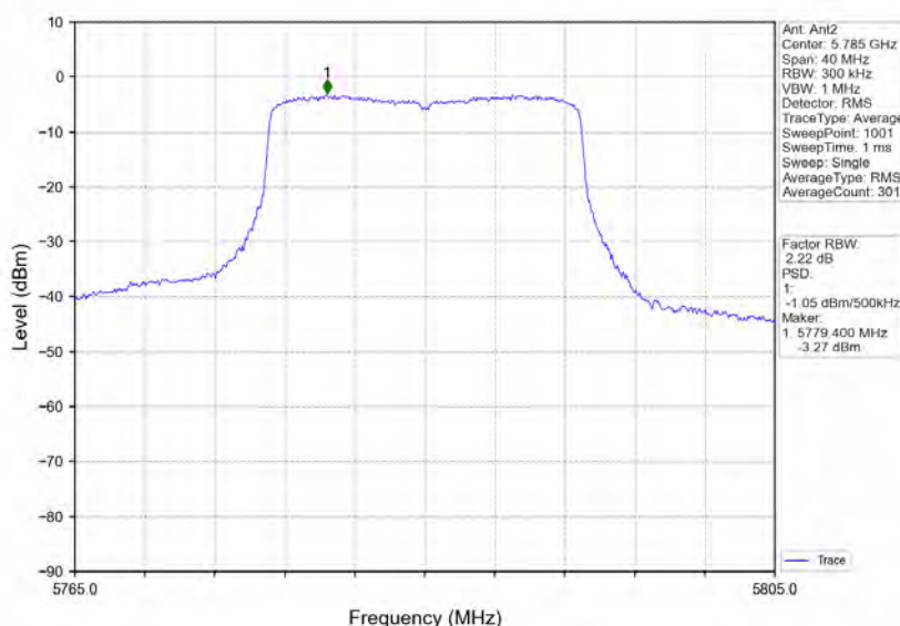
802.11n(HT20)_MCH_5785MHz_MIMO_NTNV
