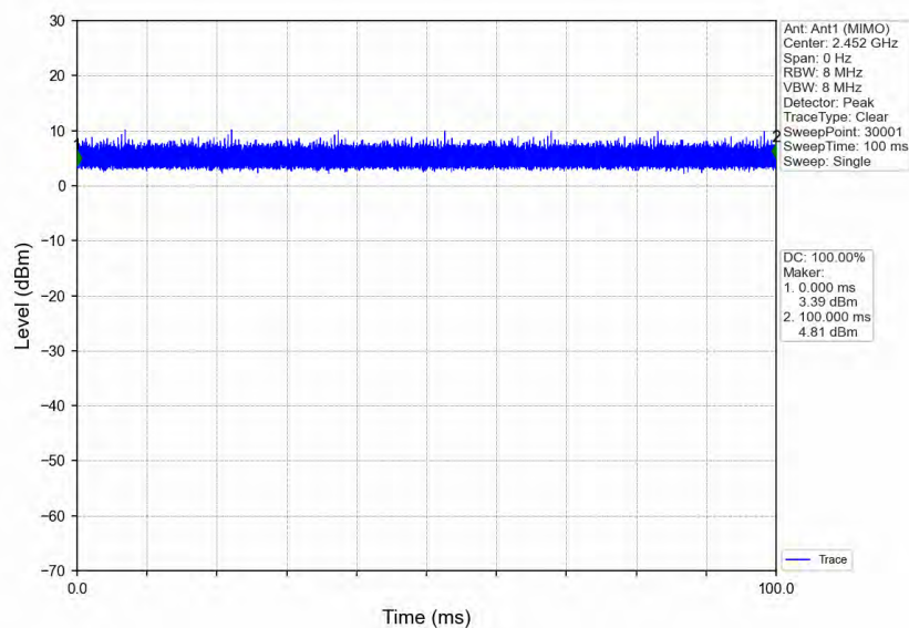
802.11n(HT40)_HCH_2452MHz_Ant1 (MIMO)_NTNV
