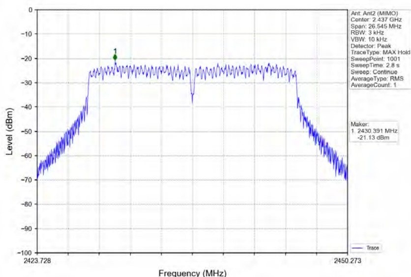
802.11n(HT20)_MCH_2437MHz_MIMO _NTNV
