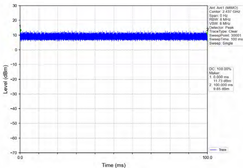
802.11n(HT20)_MCH_2437MHz_Ant1 (MIMO)_NTNV
