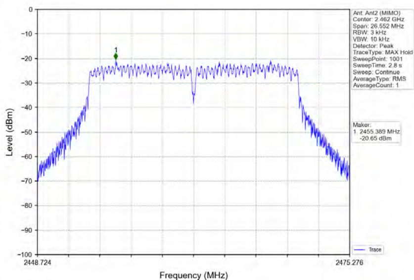
802.11n(HT20)_HCH_2462MHz_Ant2 (MIMO)_NTNV
