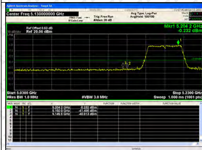
802.11ac(HT80)-5210
