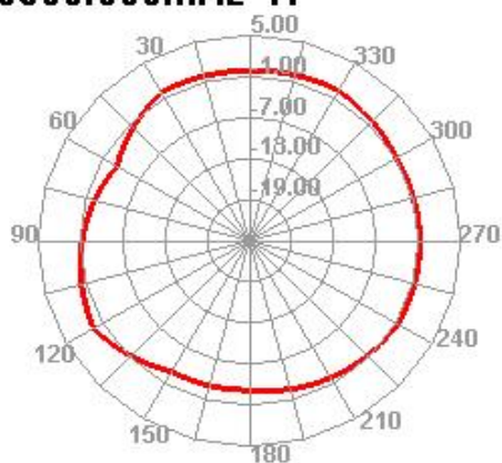
5500.000MHz H
