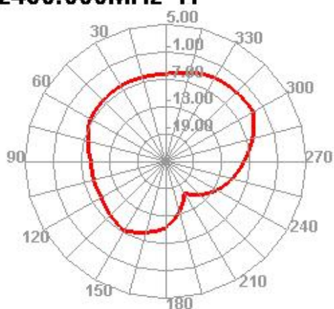
2450.000MHz H
