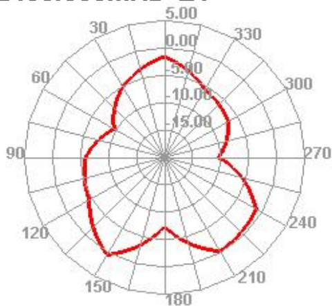
2450.000MHz E1
