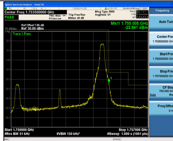
Band4 5MHz 16QAM 20375 1RB#24
