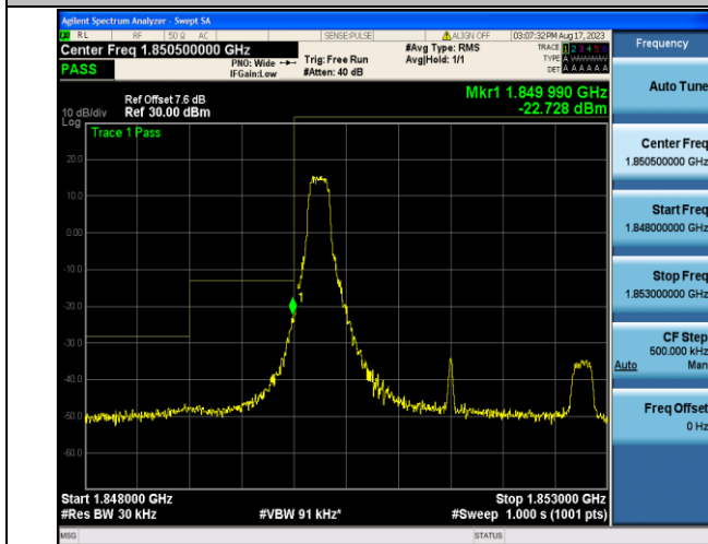
Band2_3MHz_QPSK_18615_1RB#0
