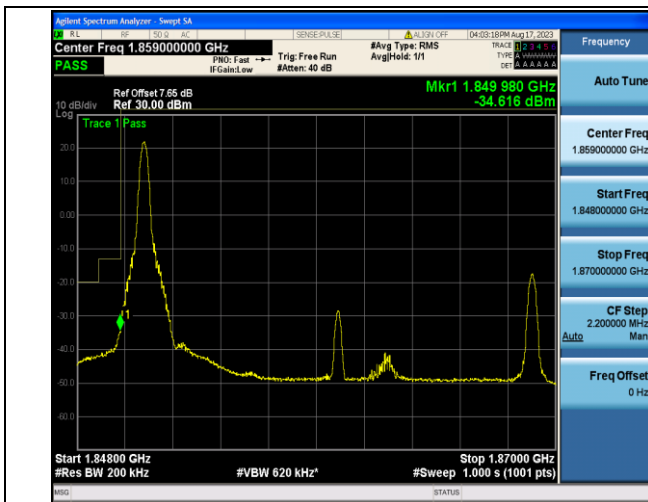
Band2_20MHz_QPSK_18700_1RB#0
