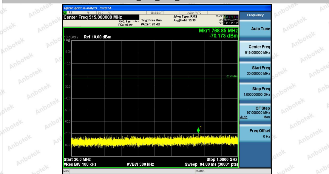
2.4_Ant1_2446_30~1000
