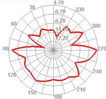
5100.000MHz E2
