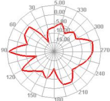
5450.000MHz E1
