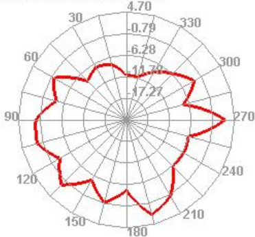
5100.000MHz E1
