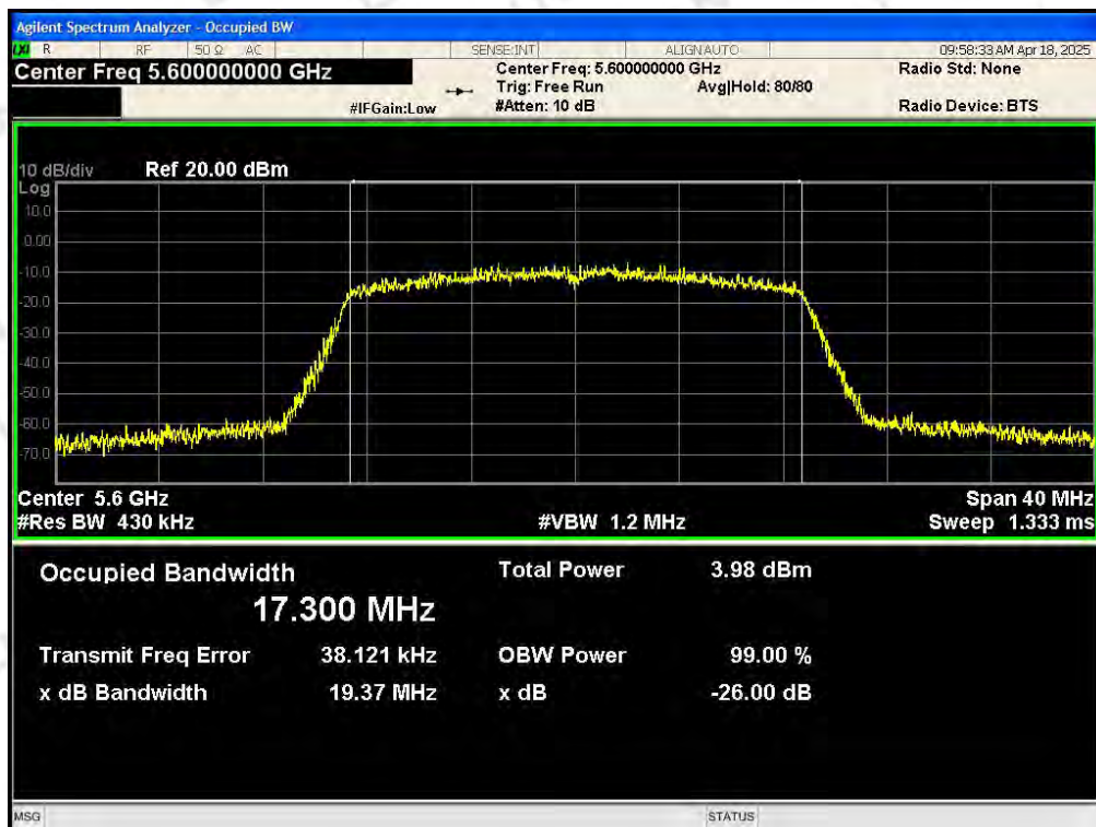
-26 dB Bandwidth NVNT 802.11ac20 5600MHz Ant0
