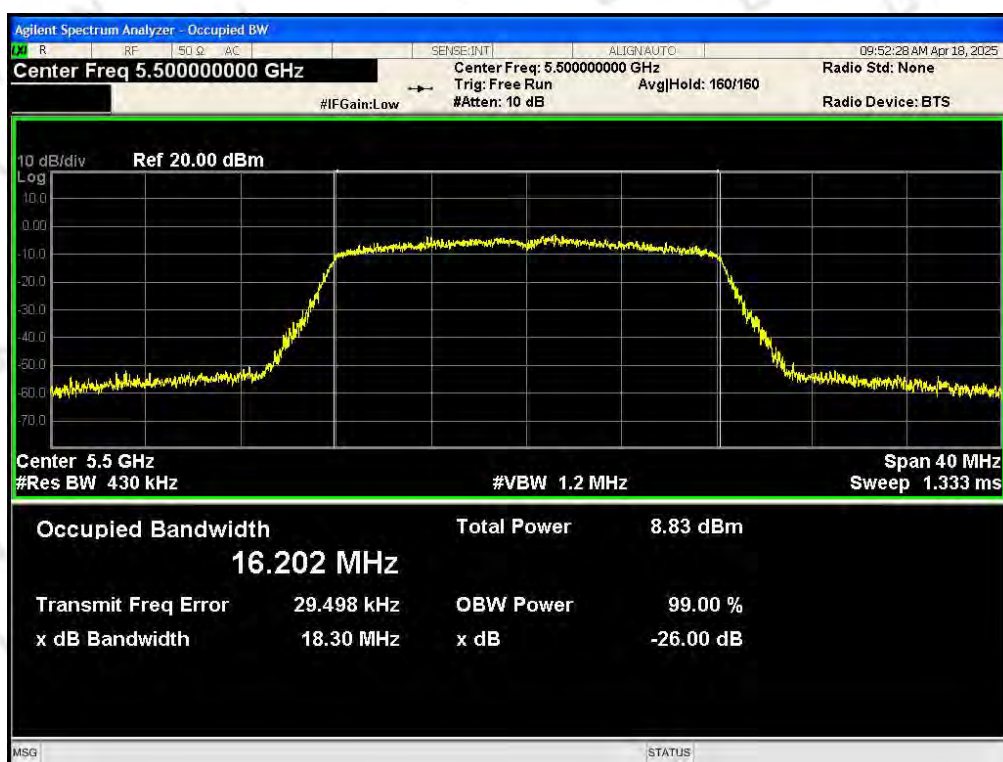
-26 dB Bandwidth NVNT 802.11a 5500MHz Ant0
