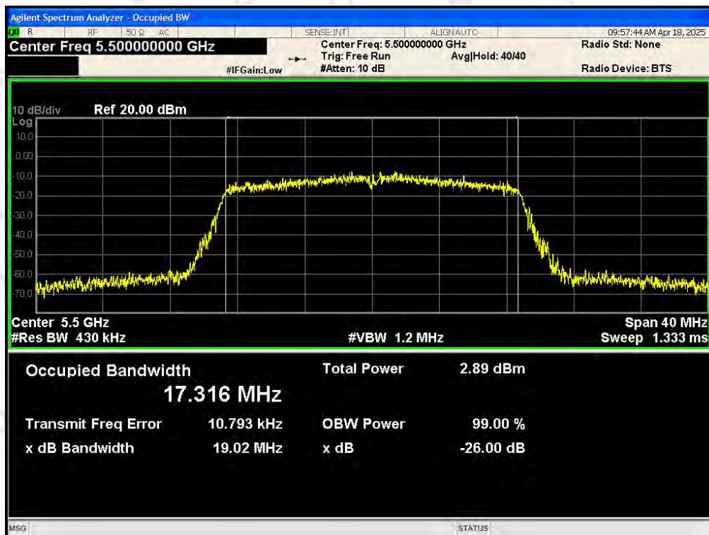
-26 dB Bandwidth NVNT 802.11ac20 5500MHz Ant0
