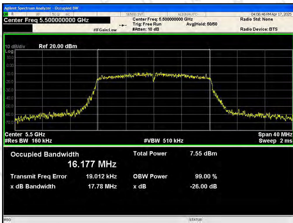
OBW NVNT 802.11a 5500MHz Ant0
