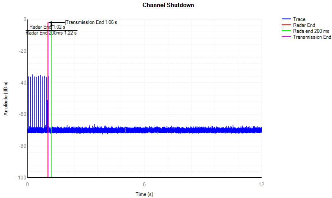
a20 5500MHz Shutdown
