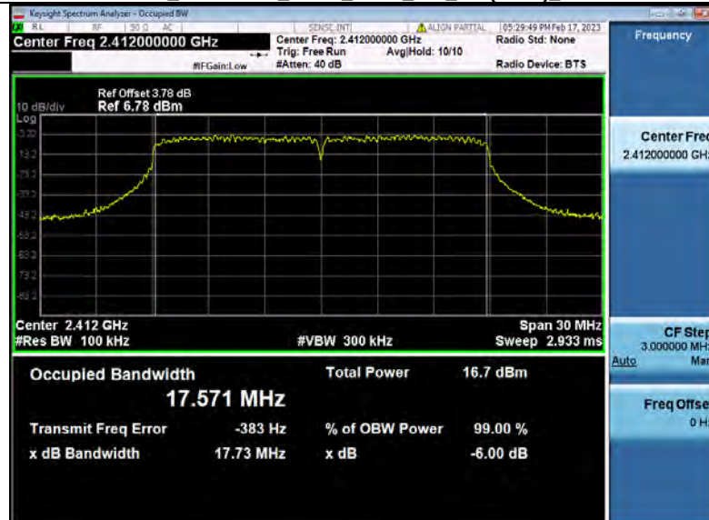
-6dB Bandwidth NVNT ANT2 802 11n(HT20) 2412
