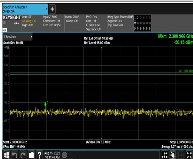
Band40-5MHz-QPSK-38750-1RB#0-Range6:2300~2305MHz
