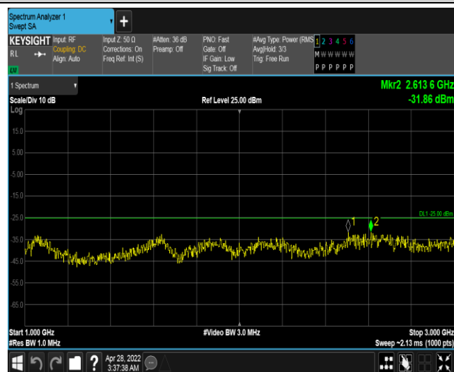
Band41-10MHz-QPSK-39700-1RB#0-Range2:1000~3000MHz
