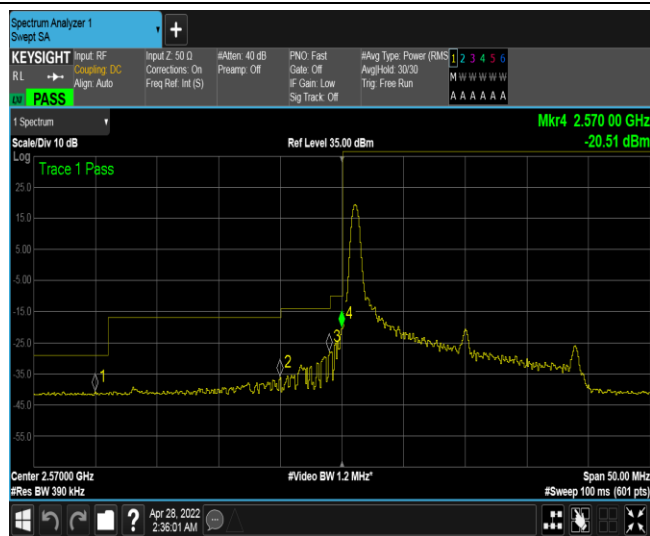
Band38-20MHz-QPSK-37850-1RB#99
