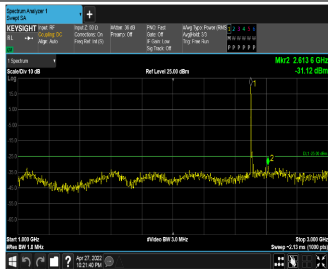
Band7-10MHz-QPSK-20800-1RB#0-Range2:1000~3000MHz
