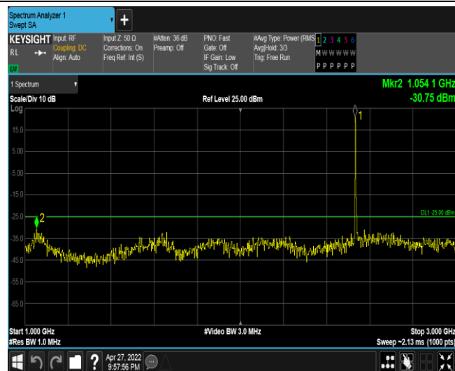
Band7-5MHz-QPSK-21100-1RB#0-Range2:1000~3000MHz
