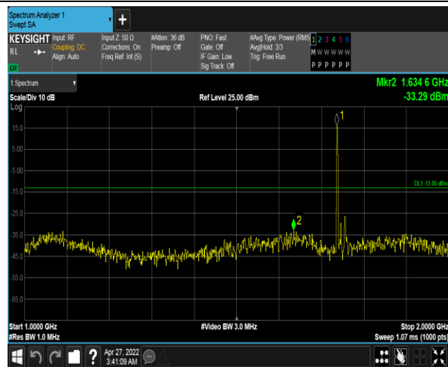
Band4-20MHz-QPSK-20300-1RB#0-Range2:1000~2000MHz
