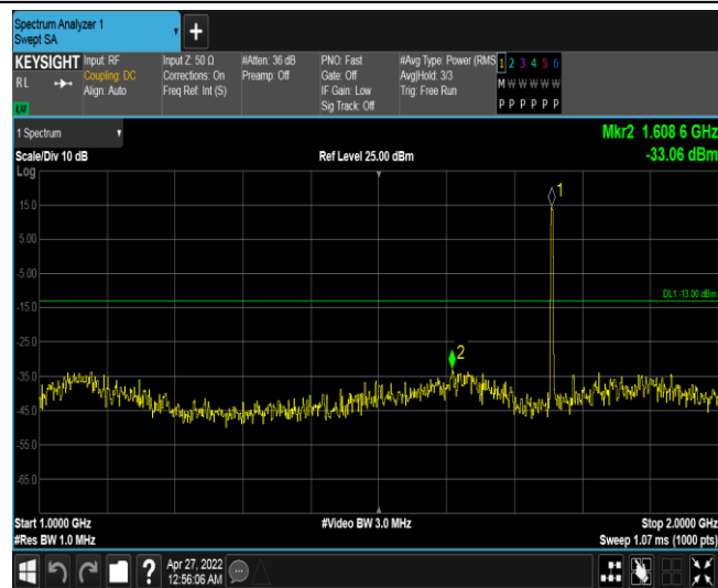
Band4-1.4MHz-QPSK-20393-1RB#0-Range2:1000~2000MHz
