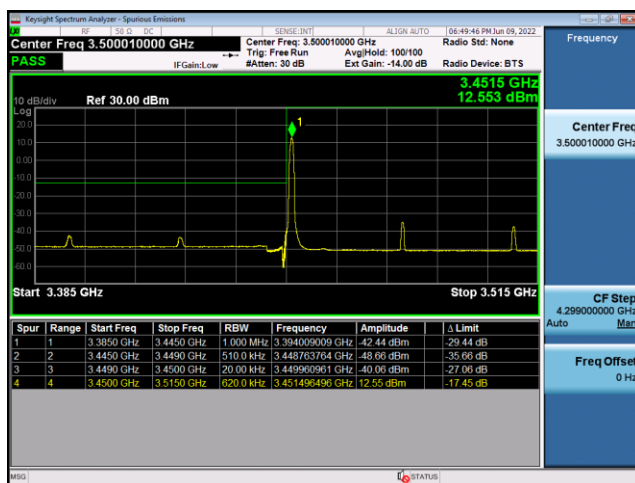
N77(60M)_CP-OFDM_QPSK_Edge_ 1RB_Left_Low_CH
