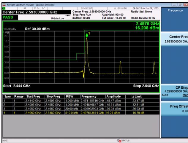
N41(50M)_CP-OFDM_QPSK_Edge_ 1RB_Left_Low_CH
