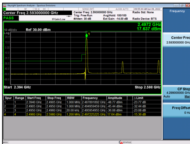
N41(100M)_CP-OFDM_QPSK_Edge_ 1RB_Left_Low_CH
