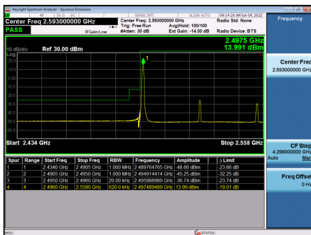
N41(60M)_CP-OFDM_QPSK_Edge_ 1RB_Left_Low_CH
