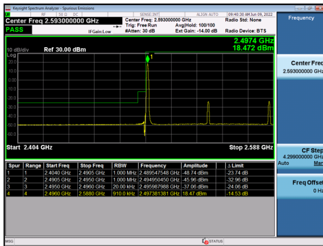
N41(90M)_CP-OFDM_QPSK_Edge_ 1RB_Left_Low_CH
