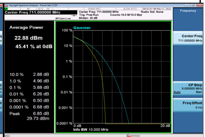
FDD17_HighRange_10MHz_711_fullRB _16QAM
