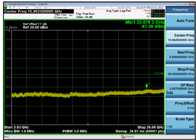
U-NII-3 ,Plot 3,5925MHz~26000MHz-802. 11ac(40MHz),5795MHz,Ant8
