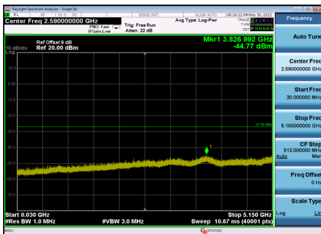
U-NII-2a ,Plot 2,30MHz~5150MHz-802.11 ac(80MHz),5290MHz,Ant9
