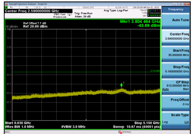
U-NII-2a ,Plot 2,30MHz~5150MHz-802.11 a(20MHz),5320MHz,Ant8
