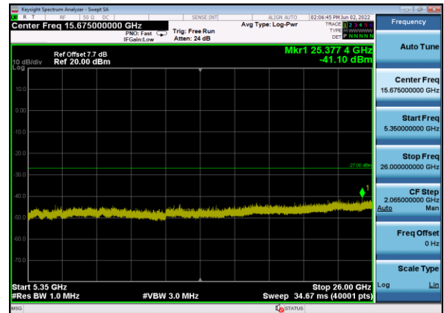
U-NII-2a ,Plot 3,5350MHz~26000MHz-802 .11ax(20MHz),5300MHz,Ant8
