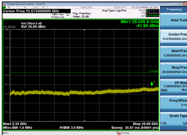
U-NII-2a ,Plot 3,5350MHz~26000MHz-802 .11ax(20MHz),5300MHz,Ant9
