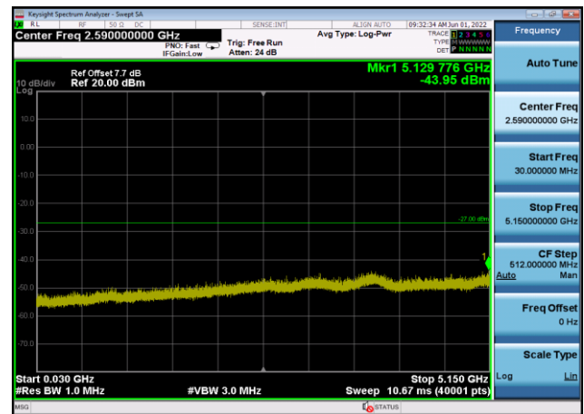
U-NII-2a ,Plot 2,30MHz~5150MHz-802.11 ac(160MHz),5250MHz,Ant8
