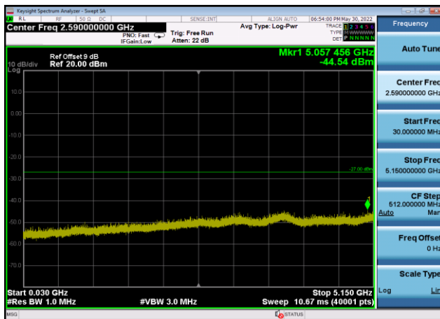
U-NII-2a ,Plot 2,30MHz~5150MHz-802.11 ac(20MHz),5300MHz,Ant9
