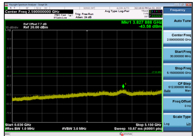
U-NII-2a ,Plot 2,30MHz~5150MHz-802.11 ax(40MHz),5270MHz,Ant8
