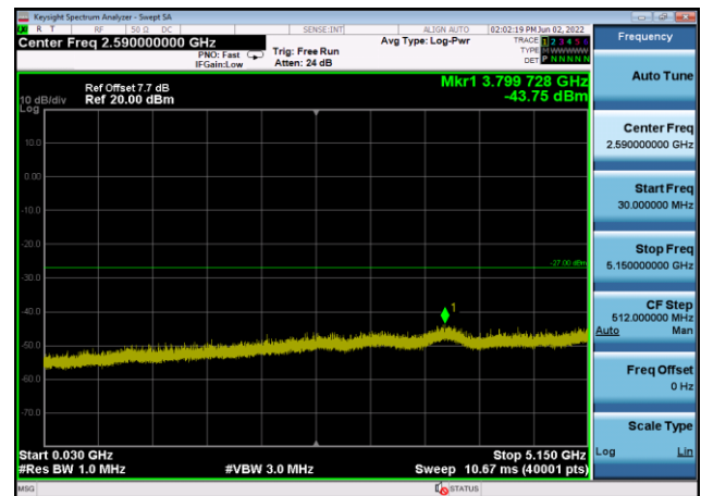
U-NII-2a ,Plot 2,30MHz~5150MHz-802.11 ac(20MHz),5300MHz,Ant8
