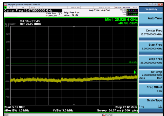
U-NII-2a ,Plot 3,5350MHz~26000MHz-802 .11ac(40MHz),5270MHz,Ant8
