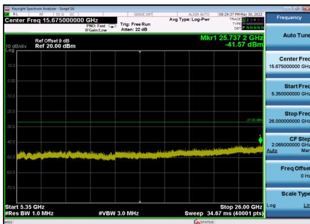
U-NII-2a ,Plot 3,5350MHz~26000MHz-802 .11ax(80MHz),5290MHz,Ant9
