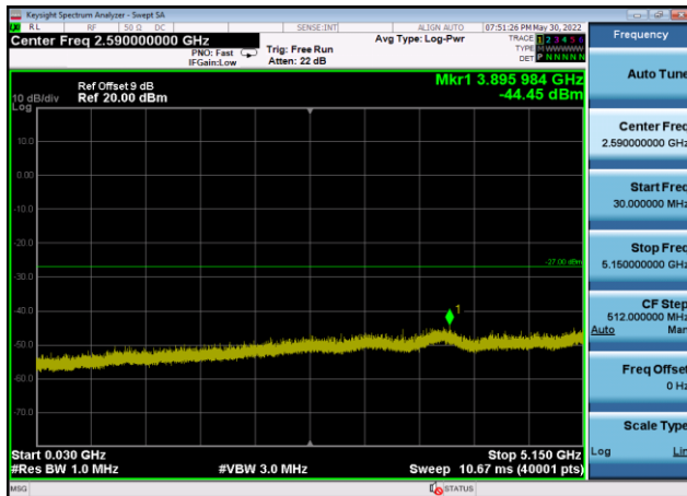
U-NII-2a ,Plot 2,30MHz~5150MHz-802.11 ac(40MHz),5310MHz,Ant9
