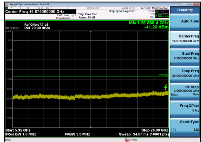
U-NII-2a ,Plot 3,5350MHz~26000MHz-802 .11ac(80MHz),5290MHz,Ant8
