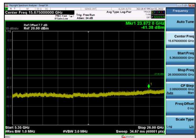
U-NII-2a ,Plot 3,5350MHz~26000MHz-802 .11ax(20MHz),5320MHz,Ant8
