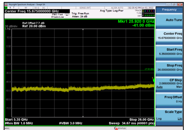
U-NII-2a ,Plot 3,5350MHz~26000MHz-802 .11ac(20MHz),5260MHz,Ant8
