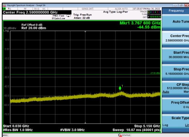
U-NII-2a ,Plot 2,30MHz~5150MHz-802.11 ax(40MHz),5310MHz,Ant9
