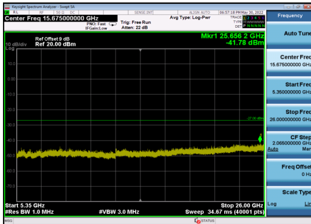
U-NII-2a ,Plot 3,5350MHz~26000MHz-802 .11ac(20MHz),5320MHz,Ant9
