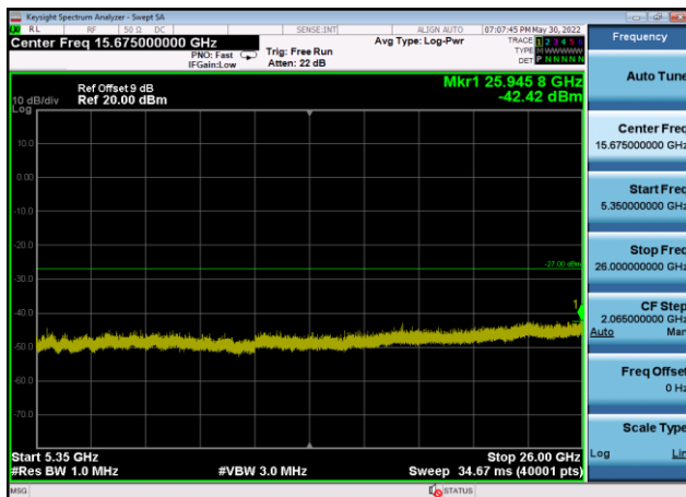
U-NII-2a ,Plot 3,5350MHz~26000MHz-802 .11ac(40MHz),5270MHz,Ant9
