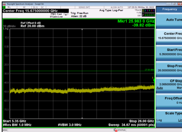
U-NII-2a ,Plot 3,5350MHz~26000MHz-802 .11ax(40MHz),5310MHz,Ant9
