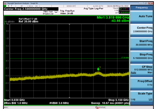
U-NII-2a ,Plot 2,30MHz~5150MHz-802.11 ac(40MHz),5310MHz,Ant8
