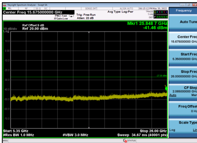
U-NII-2a ,Plot 3,5350MHz~26000MHz-802 .11a(20MHz),5300MHz,Ant9
