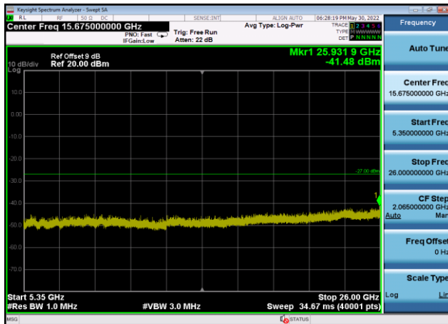
U-NII-2a ,Plot 3,5350MHz~26000MHz-802 .11ac(160MHz),5250MHz,Ant9
