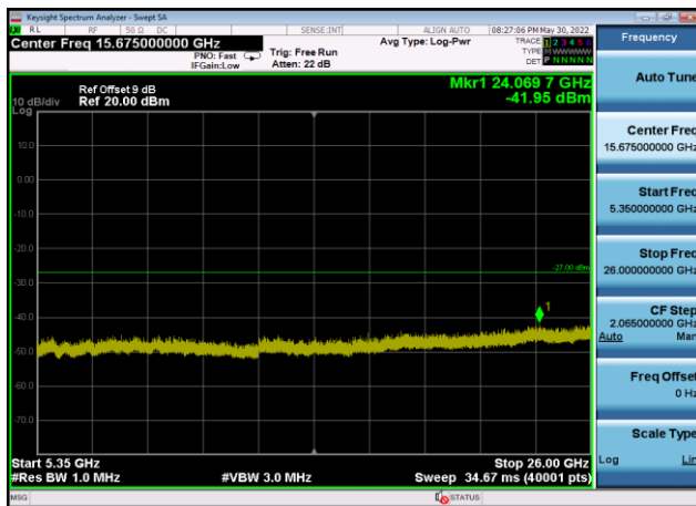
U-NII-2a ,Plot 3,5350MHz~26000MHz-802 .11ax(160MHz),5250MHz,Ant9
