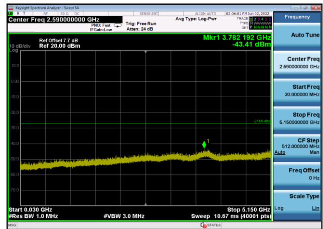
U-NII-2a ,Plot 2,30MHz~5150MHz-802.11 ax(20MHz),5300MHz,Ant8
