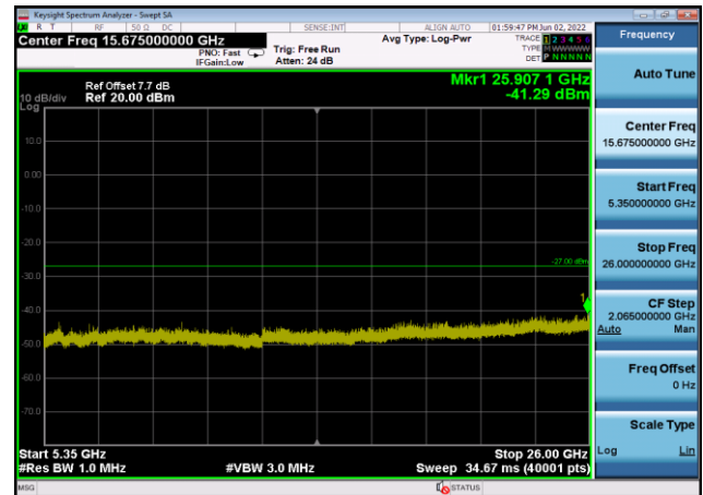
U-NII-2a ,Plot 3,5350MHz~26000MHz-802 .11ac(20MHz),5320MHz,Ant8
