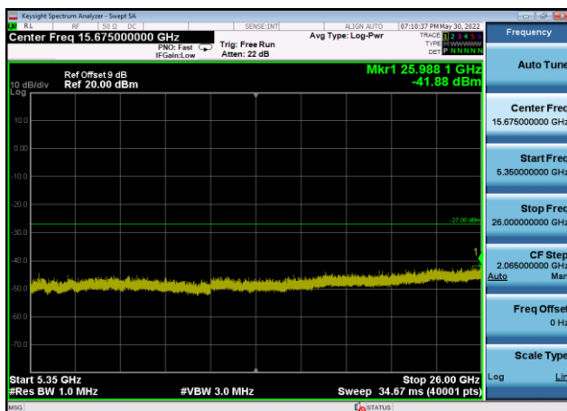
U-NII-2a ,Plot 3,5350MHz~26000MHz-802 .11ax(20MHz),5320MHz,Ant9
