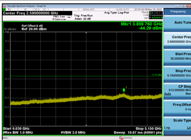
U-NII-2a ,Plot 2,30MHz~5150MHz-802.11 ac(20MHz),5320MHz,Ant9
