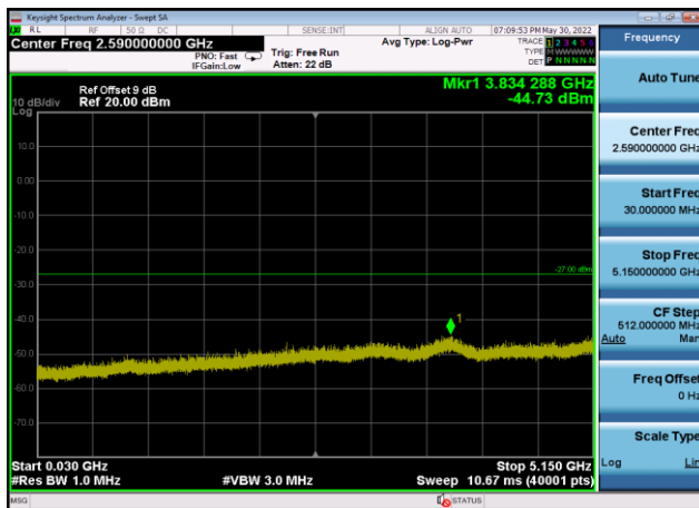
U-NII-2a ,Plot 2,30MHz~5150MHz-802.11 ax(40MHz),5270MHz,Ant9
