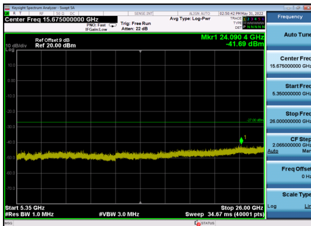
U-NII-2a ,Plot 3,5350MHz~26000MHz-802 .11ac(20MHz),5260MHz,Ant9
