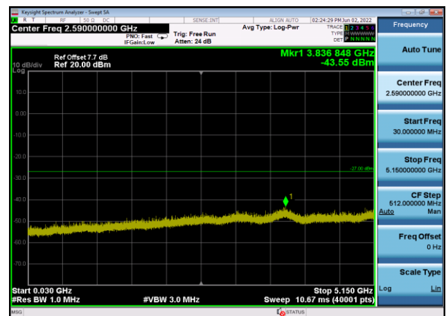
U-NII-2a ,Plot 2,30MHz~5150MHz-802.11 ax(40MHz),5310MHz,Ant8
