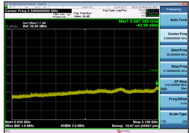
U-NII-2a ,Plot 2,30MHz~5150MHz-802.11 ax(20MHz),5260MHz,Ant8
