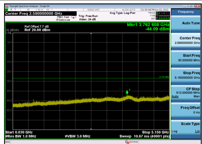
U-NII-2a ,Plot 2,30MHz~5150MHz-802.11 ac(20MHz),5320MHz,Ant8
