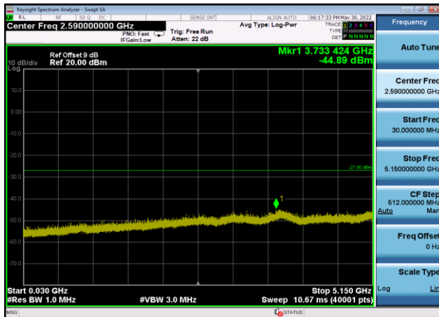
U-NII-2a ,Plot 2,30MHz~5150MHz-802.11 a(20MHz),5320MHz,Ant9
