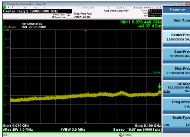
U-NII-2a ,Plot 2,30MHz~5150MHz-802.11 ax(20MHz),5260MHz,Ant9
