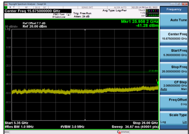
U-NII-2a ,Plot 3,5350MHz~26000MHz-802 .11ax(40MHz),5310MHz,Ant8
