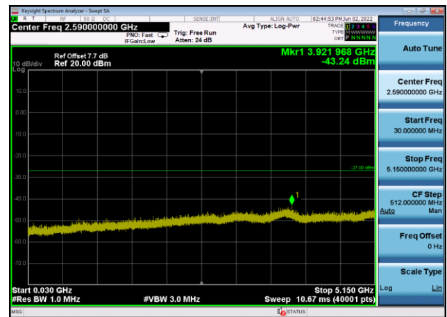
U-NII-2a ,Plot 2,30MHz~5150MHz-802.11 ac(80MHz),5290MHz,Ant8
