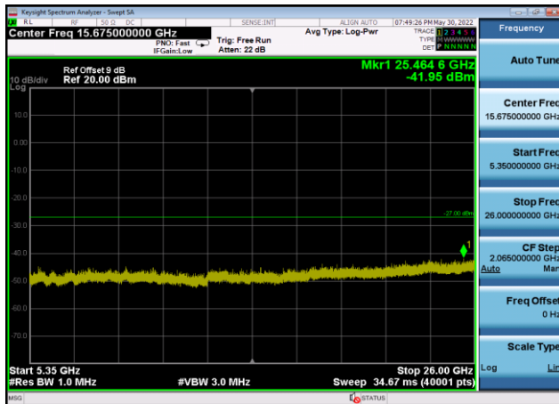
U-NII-2a ,Plot 3,5350MHz~26000MHz-802 .11ac(80MHz),5290MHz,Ant9
