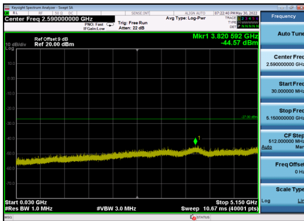
U-NII-2a ,Plot 2,30MHz~5150MHz-802.11 ax(20MHz),5300MHz,Ant9
