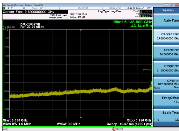
U-NII-2a ,Plot 2,30MHz~5150MHz-802.11 ac(160MHz),5250MHz,Ant9
