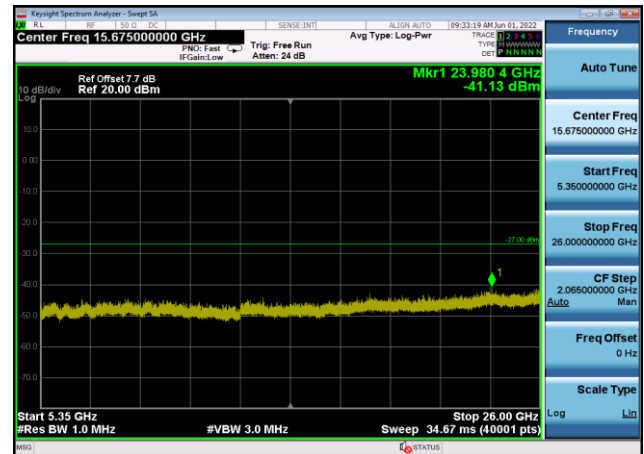
U-NII-2a ,Plot 3,5350MHz~26000MHz-802 .11ac(160MHz),5250MHz,Ant8
