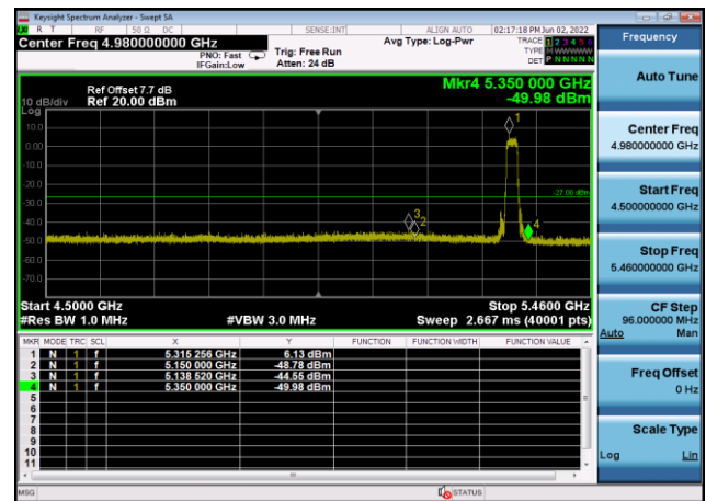
U-NII-2a ,Plot 1,Band Edge-802.11ax(4 0MHz),5270MHz,Ant8
