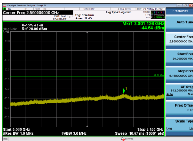
U-NII-2a ,Plot 2,30MHz~5150MHz-802.11 n(40MHz),5270MHz,Ant9
