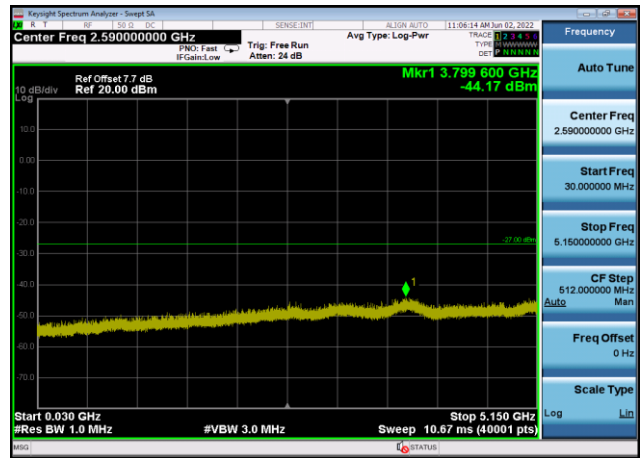
U-NII-2a ,Plot 2,30MHz~5150MHz-802.11 n(20MHz),5300MHz,Ant8
