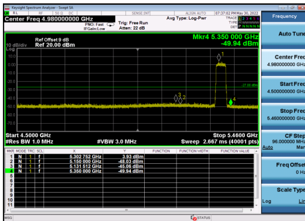
U-NII-2a ,Plot 1,Band Edge-802.11ax(8 0MHz),5290MHz,Ant9
