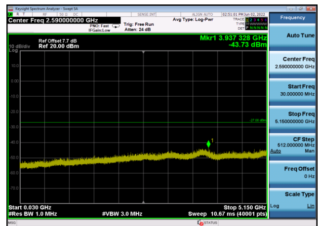
U-NII-2a ,Plot 2,30MHz~5150MHz-802.11 n(40MHz),5270MHz,Ant8
