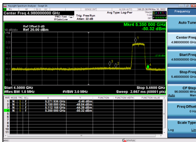
U-NII-2a ,Plot 1,Band Edge-802.11ax(1 60MHz),5250MHz,Ant9
