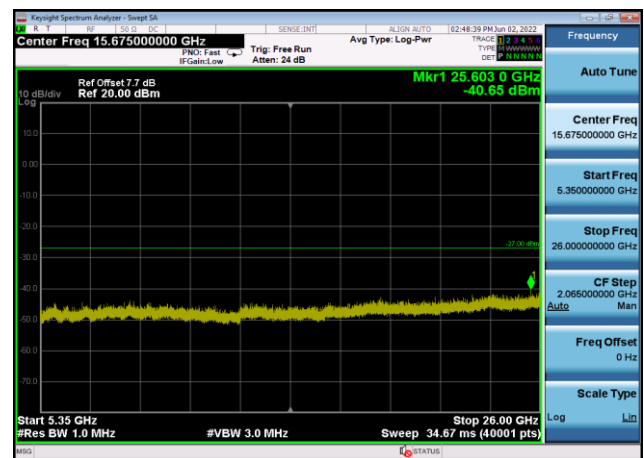
U-NII-2a ,Plot 3,5350MHz~26000MHz-802 .11n(40MHz),5310MHz,Ant8
