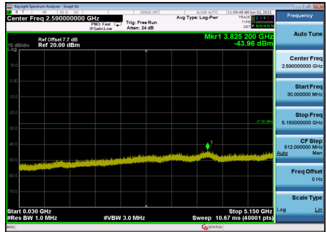
U-NII-2a ,Plot 2,30MHz~5150MHz-802.11 n(20MHz),5320MHz,Ant8
