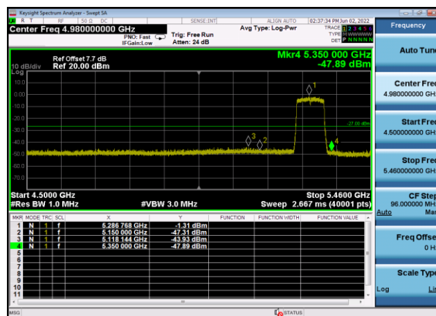
U-NII-2a ,Plot 1,Band Edge-802.11ax(1 60MHz),5250MHz,Ant8
