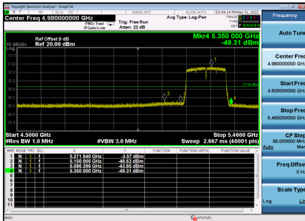
U-NII-2a ,Plot 1,Band Edge-802.11ac(2 0MHz),5260MHz,Ant9
