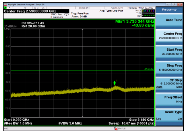
U-NII-2a ,Plot 2,30MHz~5150MHz-802.11 n(20MHz),5320MHz,Ant8
