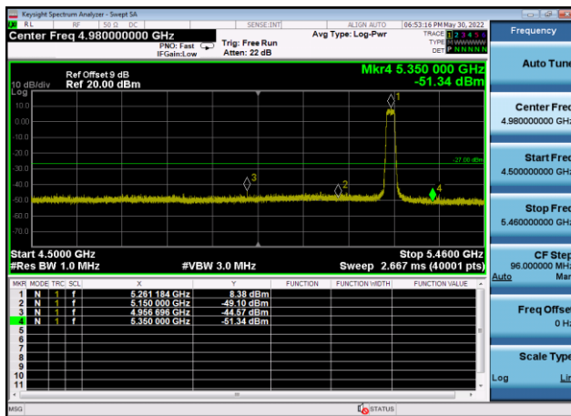
U-NII-2a ,Plot 1,Band Edge-802.11ac(2 0MHz),5300MHz,Ant9
