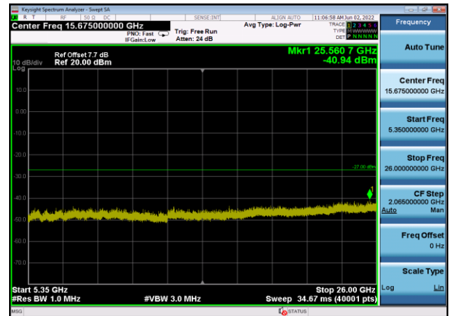
U-NII-2a ,Plot 3,5350MHz~26000MHz-802 .11n(20MHz),5300MHz,Ant8
