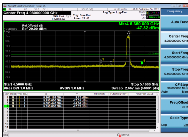
U-NII-2a ,Plot 1,Band Edge-802.11ax(2 0MHz),5260MHz,Ant9
