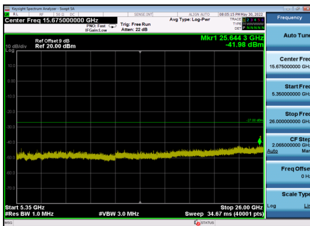
U-NII-2a ,Plot 3,5350MHz~26000MHz-802 .11n(40MHz),5310MHz,Ant9
