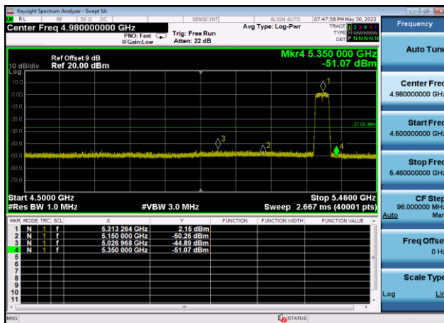
U-NII-2a ,Plot 1,Band Edge-802.11ac(4 0MHz),5310MHz,Ant9
