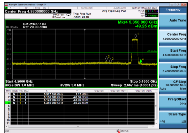
U-NII-2a ,Plot 1,Band Edge-802.11ac(4 0MHz),5310MHz,Ant8
