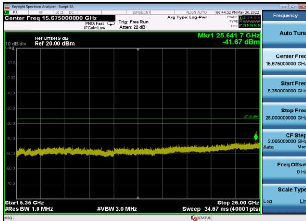
U-NII-2a ,Plot 3,5350MHz~26000MHz-802 .11n(20MHz),5300MHz,Ant9
