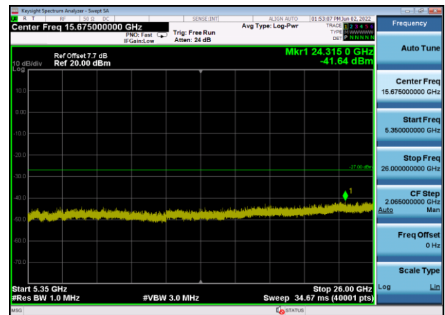
U-NII-2a ,Plot 3,5350MHz~26000MHz-802 .11n(20MHz),5320MHz,Ant8
