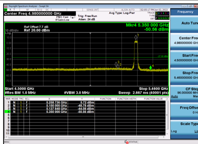
U-NII-2a ,Plot 1,Band Edge-802.11ax(2 0MHz),5260MHz,Ant8
