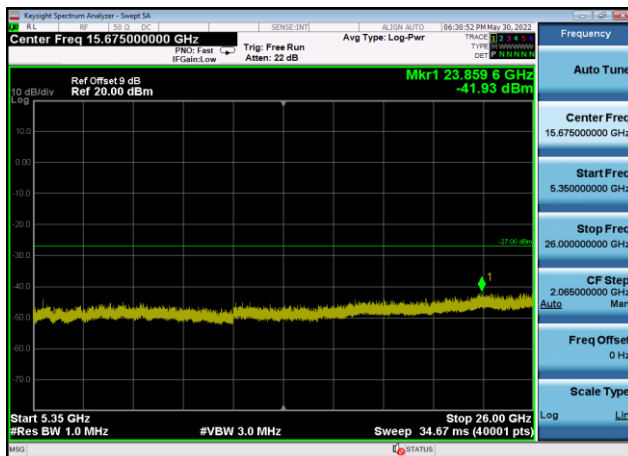
U-NII-2a ,Plot 3,5350MHz~26000MHz-802 .11n(20MHz),5320MHz,Ant9
