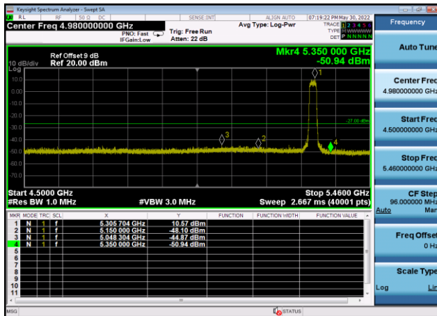
U-NII-2a ,Plot 1,Band Edge-802.11ax(2 0MHz),5320MHz,Ant9
