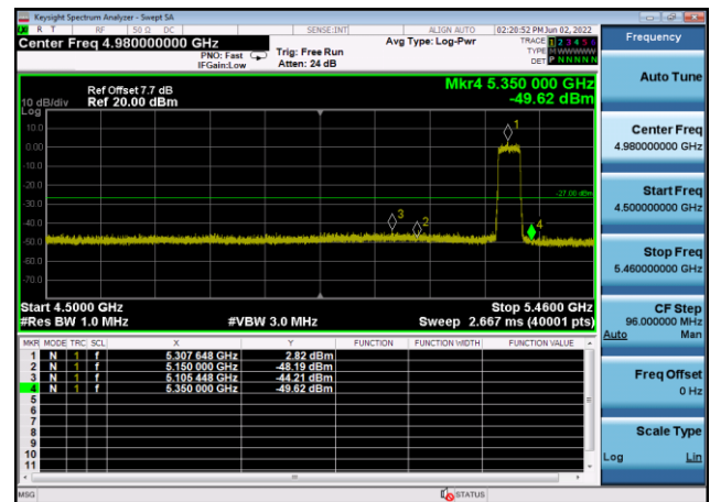
U-NII-2a ,Plot 1,Band Edge-802.11ax(8 0MHz),5290MHz,Ant8
