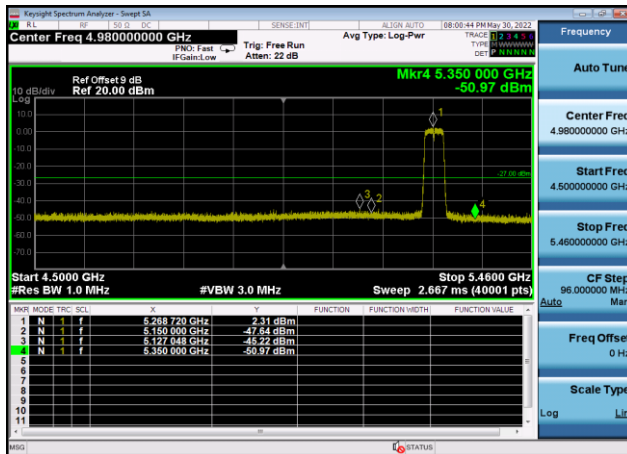
U-NII-2a ,Plot 1,Band Edge-802.11n(40 MHz),5310MHz,Ant9
