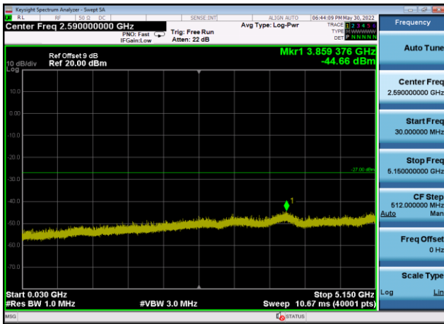
U-NII-2a ,Plot 2,30MHz~5150MHz-802.11 n(20MHz),5300MHz,Ant9
