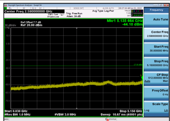
U-NII-2a ,Plot 2,30MHz~5150MHz-802.11 a(20MHz),5260MHz,Ant8
