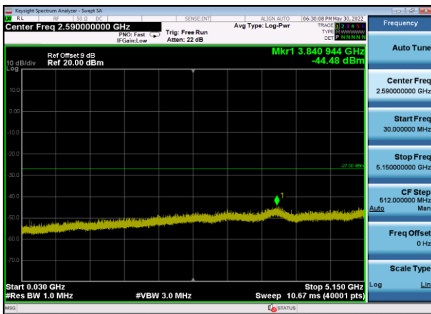
U-NII-2a ,Plot 2,30MHz~5150MHz-802.11 n(20MHz),5320MHz,Ant9
