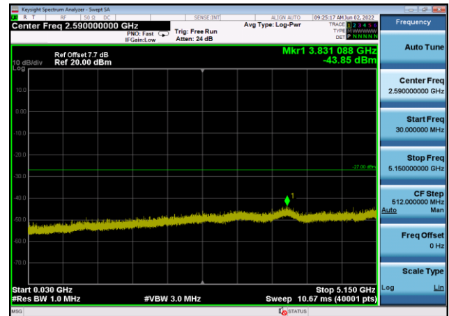
U-NII-1 ,Plot 2,30MHz~5150MHz-802.11a c(20MHz),5220MHz,Ant8
