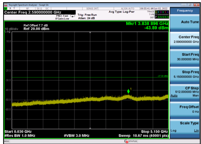
U-NII-1 ,Plot 2,30MHz~5150MHz-802.11a x(80MHz),5210MHz,Ant8
