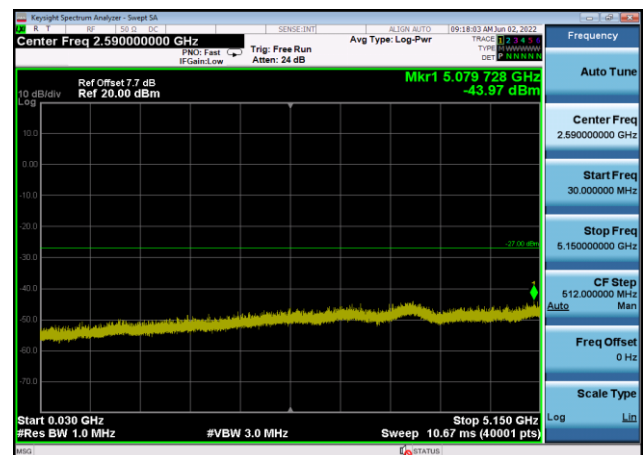
U-NII-1 ,Plot 2,30MHz~5150MHz-802.11a c(20MHz),5240MHz,Ant8
