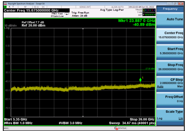
U-NII-1 ,Plot 3,5350MHz~26000MHz-802. 11ac(20MHz),5240MHz,Ant8
