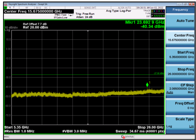
U-NII-1 ,Plot 3,5350MHz~26000MHz-802. 11ax(20MHz),5220MHz,Ant8
