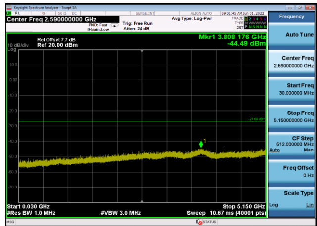
U-NII-1 ,Plot 2,30MHz~5150MHz-802.11a (20MHz),5240MHz,Ant8
