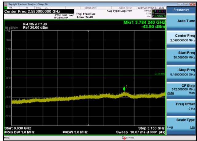
U-NII-1 ,Plot 2,30MHz~5150MHz-802.11a (20MHz),5220MHz,Ant8
