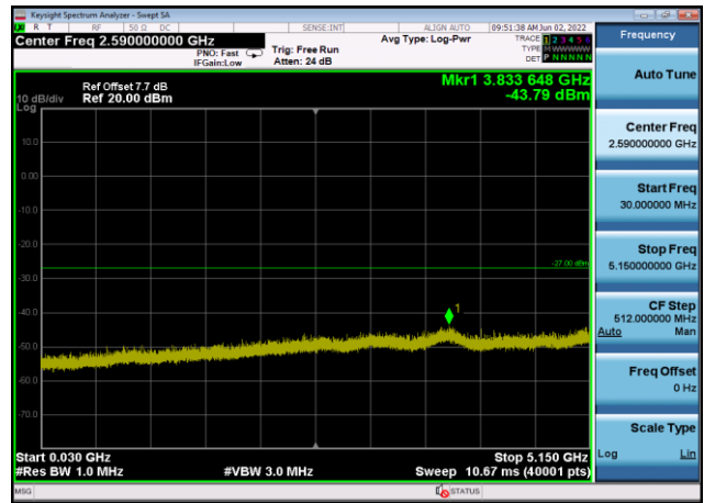
U-NII-1 ,Plot 2,30MHz~5150MHz-802.11a x(40MHz),5230MHz,Ant8
