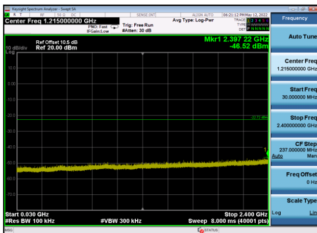
,Plot 3,30MHz~2400MHz-802.11ax(HE40) ,2452MHz,Ant9
