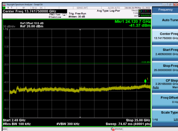
,Plot 4,2483.5MHz~25000MHz-802.11ax(H T20),2437MHz,Ant9
