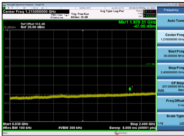
,Plot 3,30MHz~2400MHz-802.11ax(HE20) ,2462MHz,Ant9
