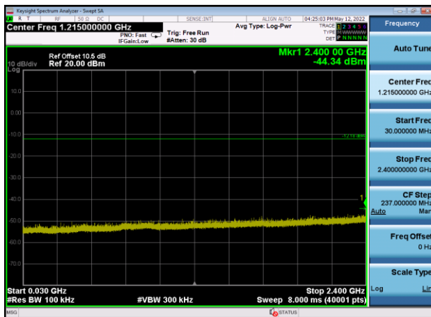
,Plot 3,30MHz~2400MHz-802.11b,2437MHz
