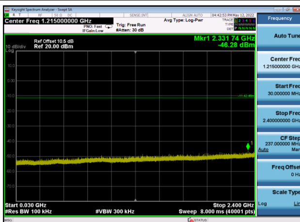
,Plot 3,30MHz~2400MHz-802.11b,2462MHz
