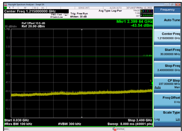
,Plot 3,30MHz~2400MHz-802.11b,2437MHz
