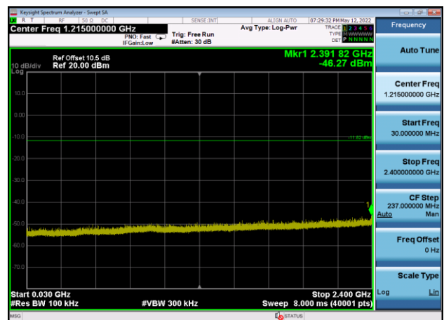
,Plot 3,30MHz~2400MHz-802.11b,2462MHz
