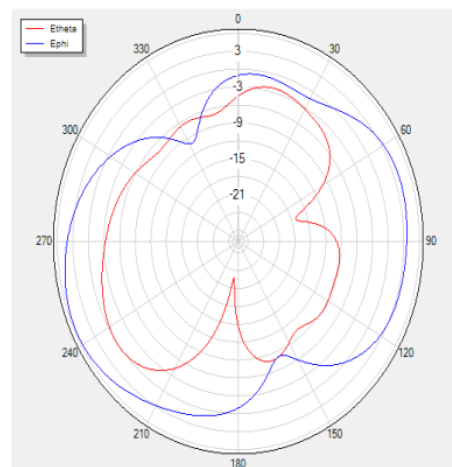
H Theta=90 freq=2400MHz
