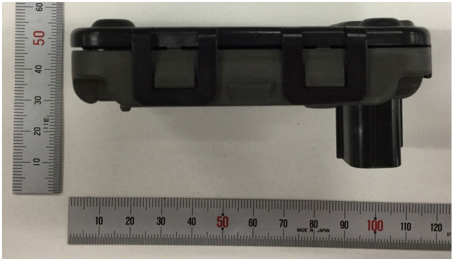
Top
