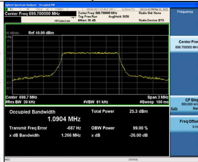
QPSK
